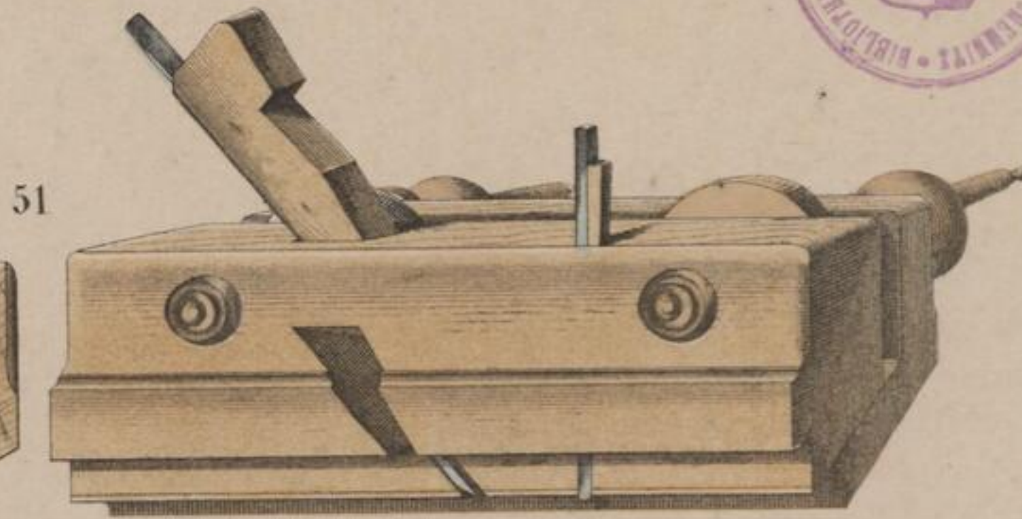
Zahnleistenhobel zum verstellen.
