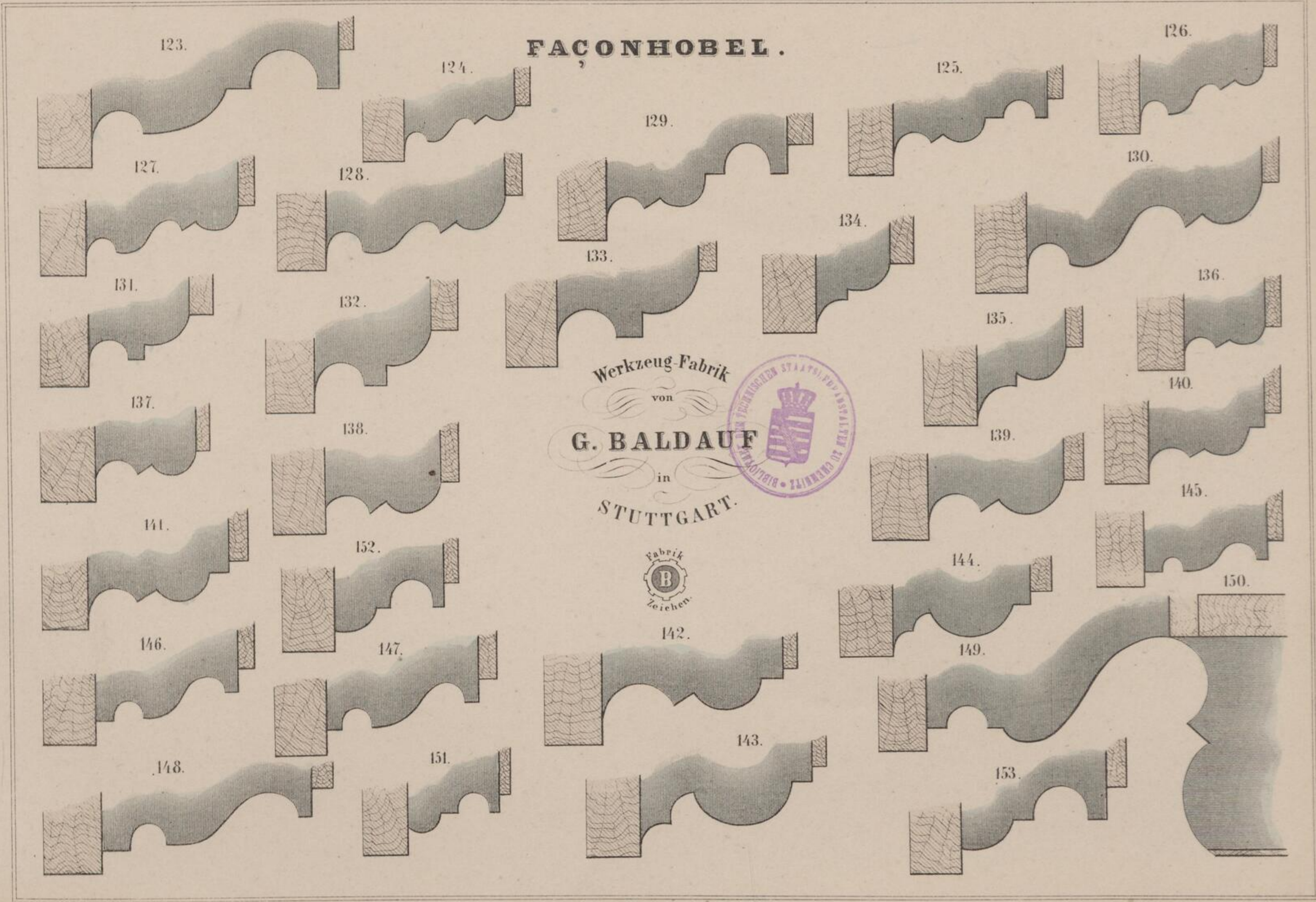
Querschnitt in natürlicher Grösse.
