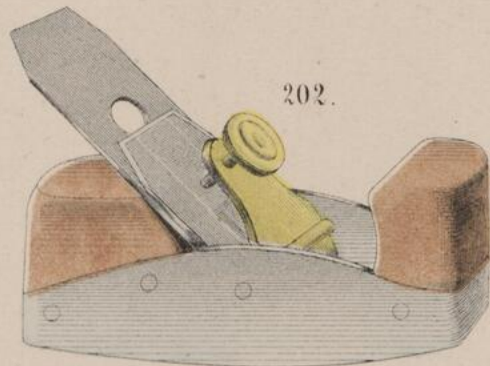
202. Doppelhobel mit Schraube.
