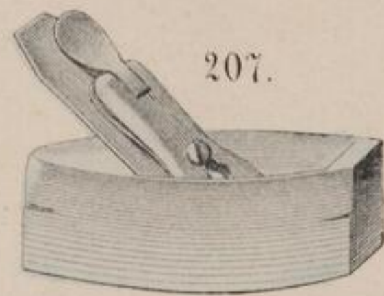
207. Putzhobel mit excentrischer Klappenvorrichtung.
