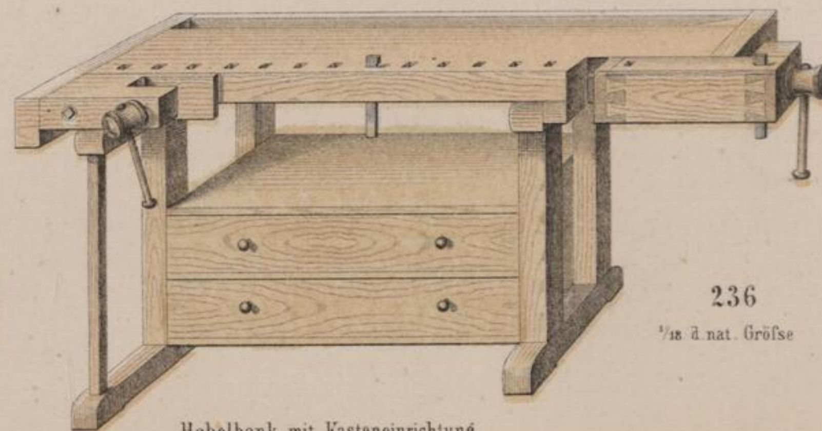
Hobelbank mit Kasteneinrichtung
