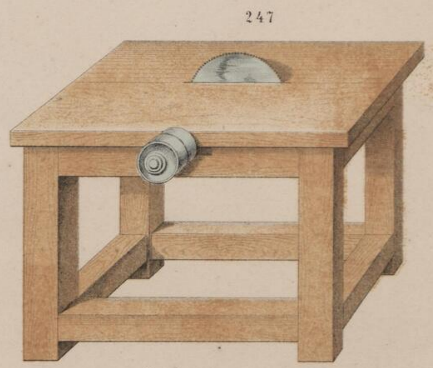
Circularsäge 1/12 d. nat. Größe
