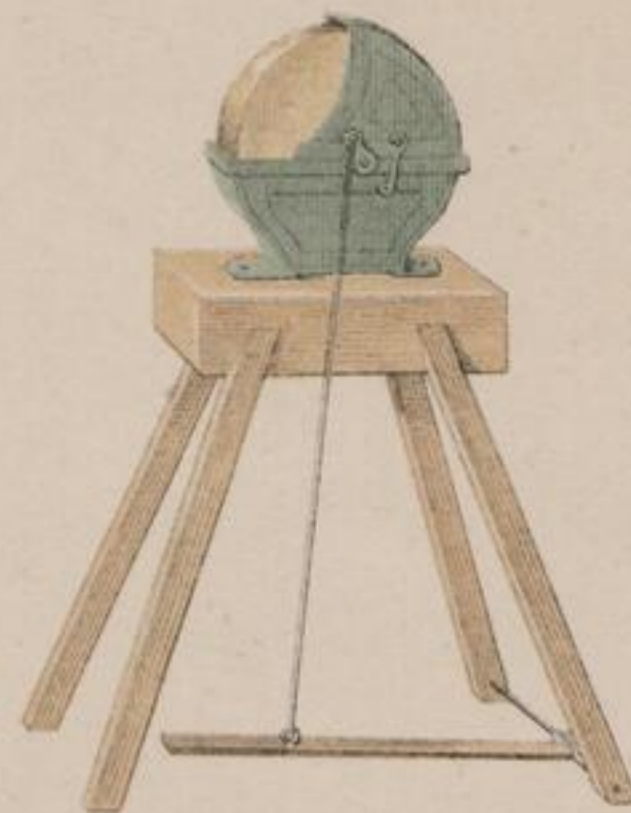
Schleifmaschine N° 5 zum treten.
