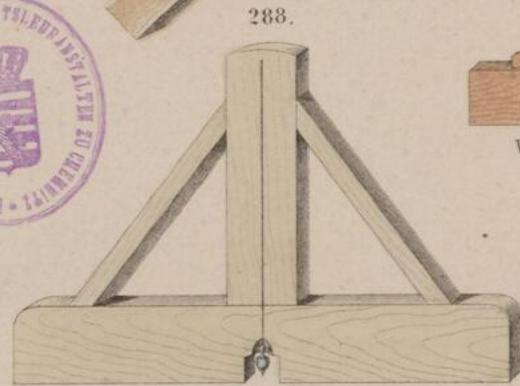
288 Bleiwaage mit Senkel. 1/8 nat. Gr.
