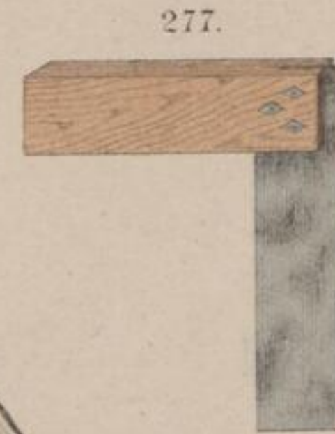
277 Winkelhacken mit Stahlschiene. 1/5 nat. Gr.
