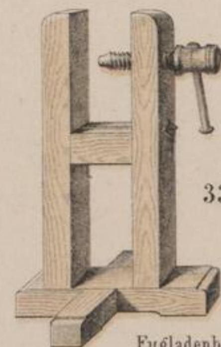
Fugladenbock 1/18 d. nat. Gr.
