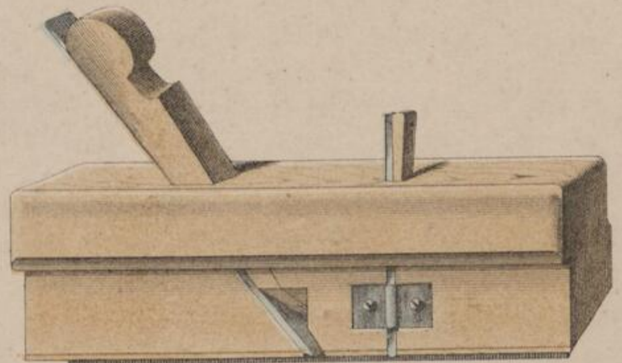
Grathhobel zum verstellen mit Messing-Anschlag.
