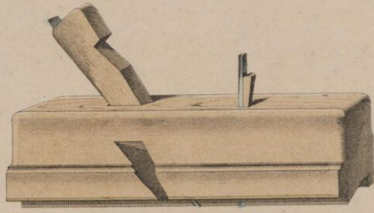
Zahnleistenhobel fest.
