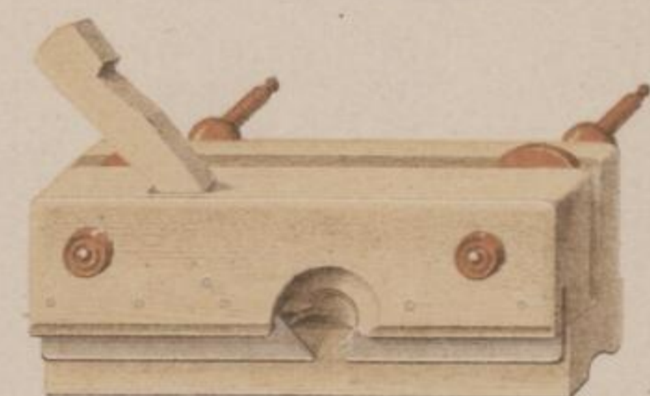
Für Glaser
