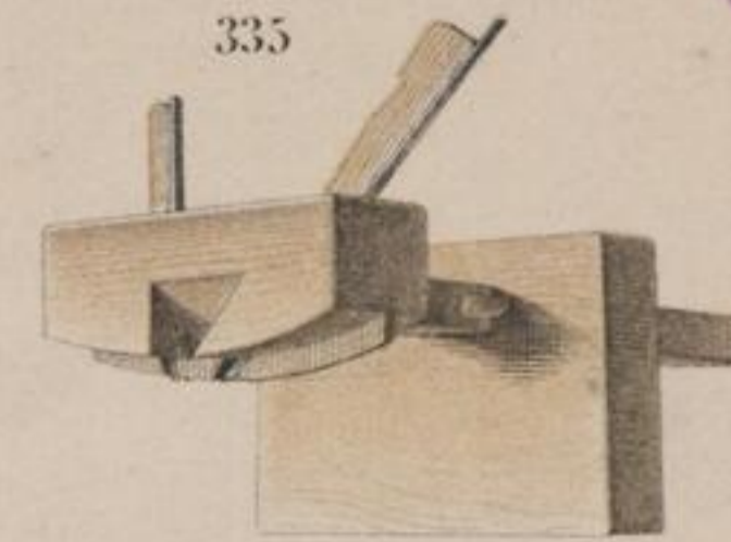
Kleiner Gargelkamm mit 1 Hobel
