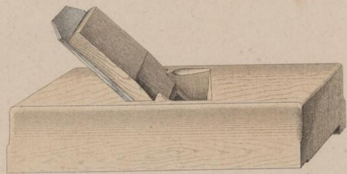
Doppelt fest.
