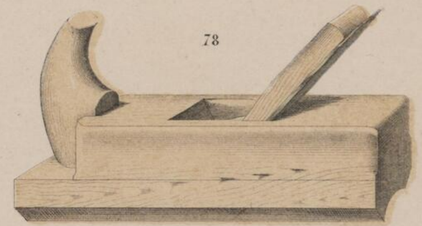
Rundstabhobel mit Nase. 1/3 nat. Gr.
