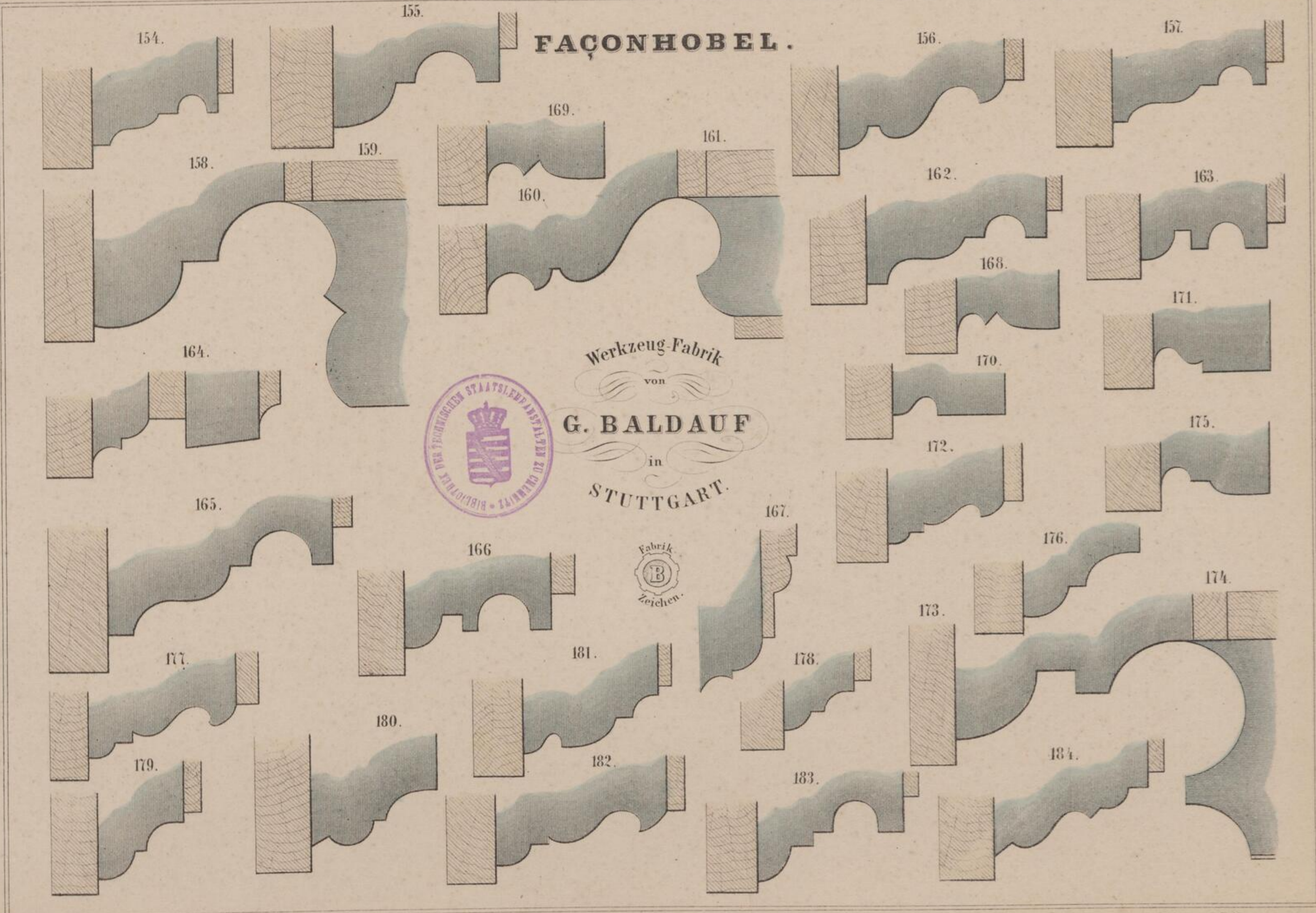
Querschnitt in natürlicher Grösse.
