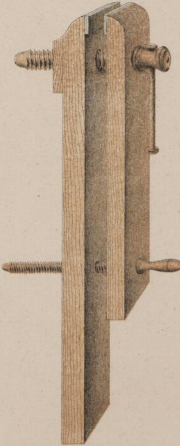
Feilkluppe. 1/8 nat. Grösse.
