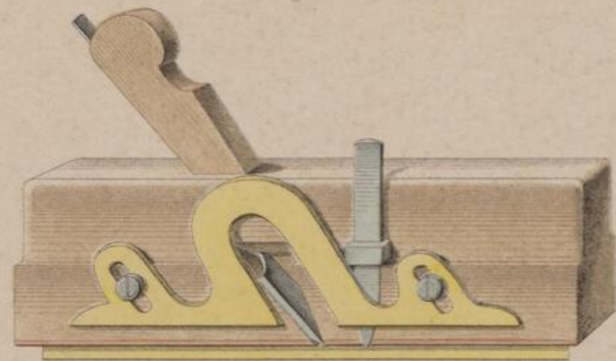
Falzhobel zum verstellen
