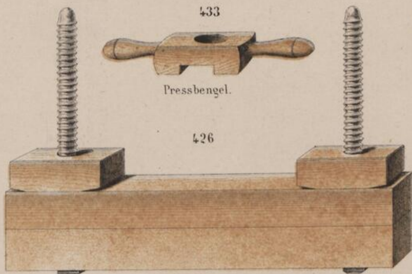
Handpresse.
