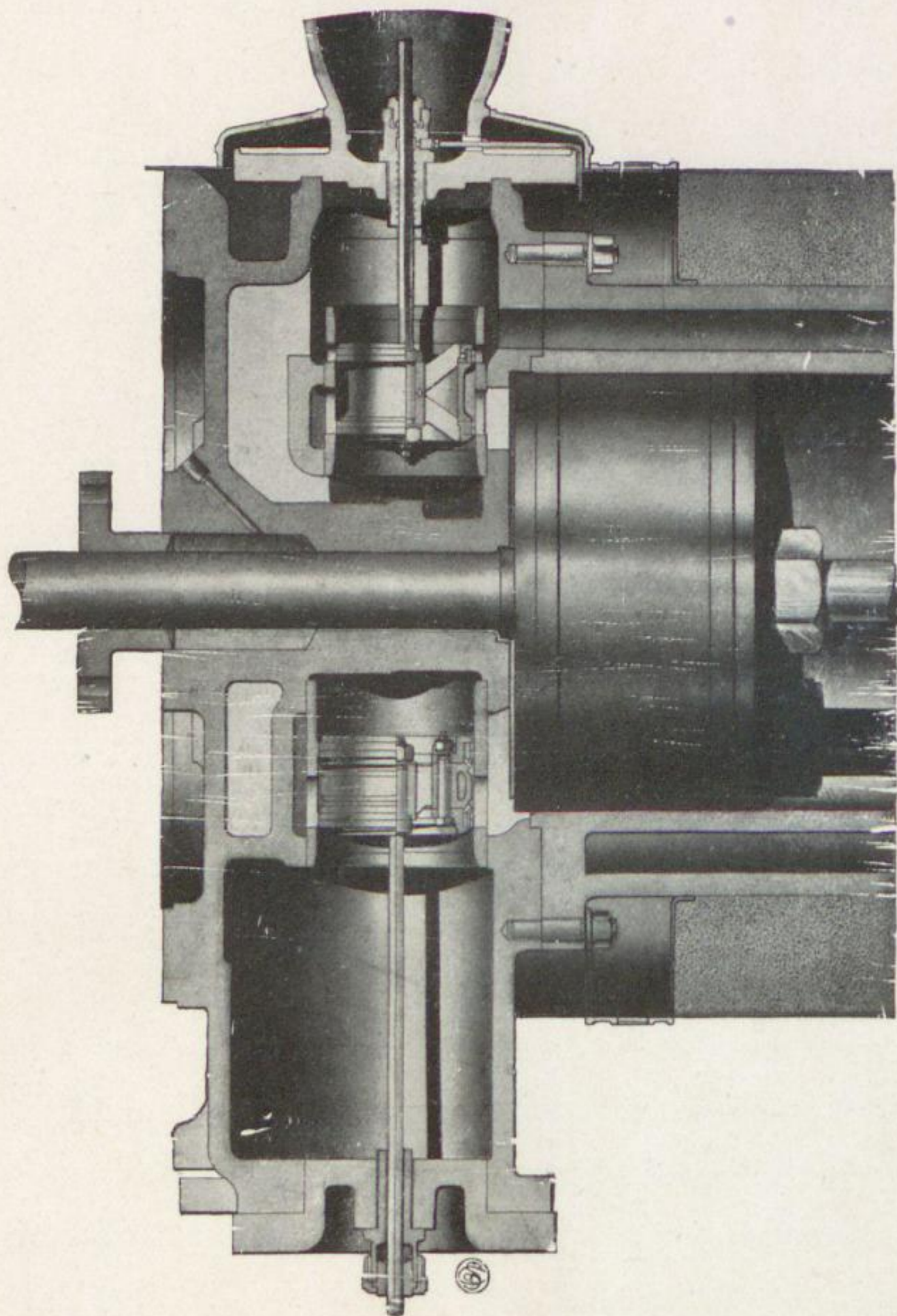
Schnitt durch den Zylinderkopf einer Kerchovedampfmaschine.
