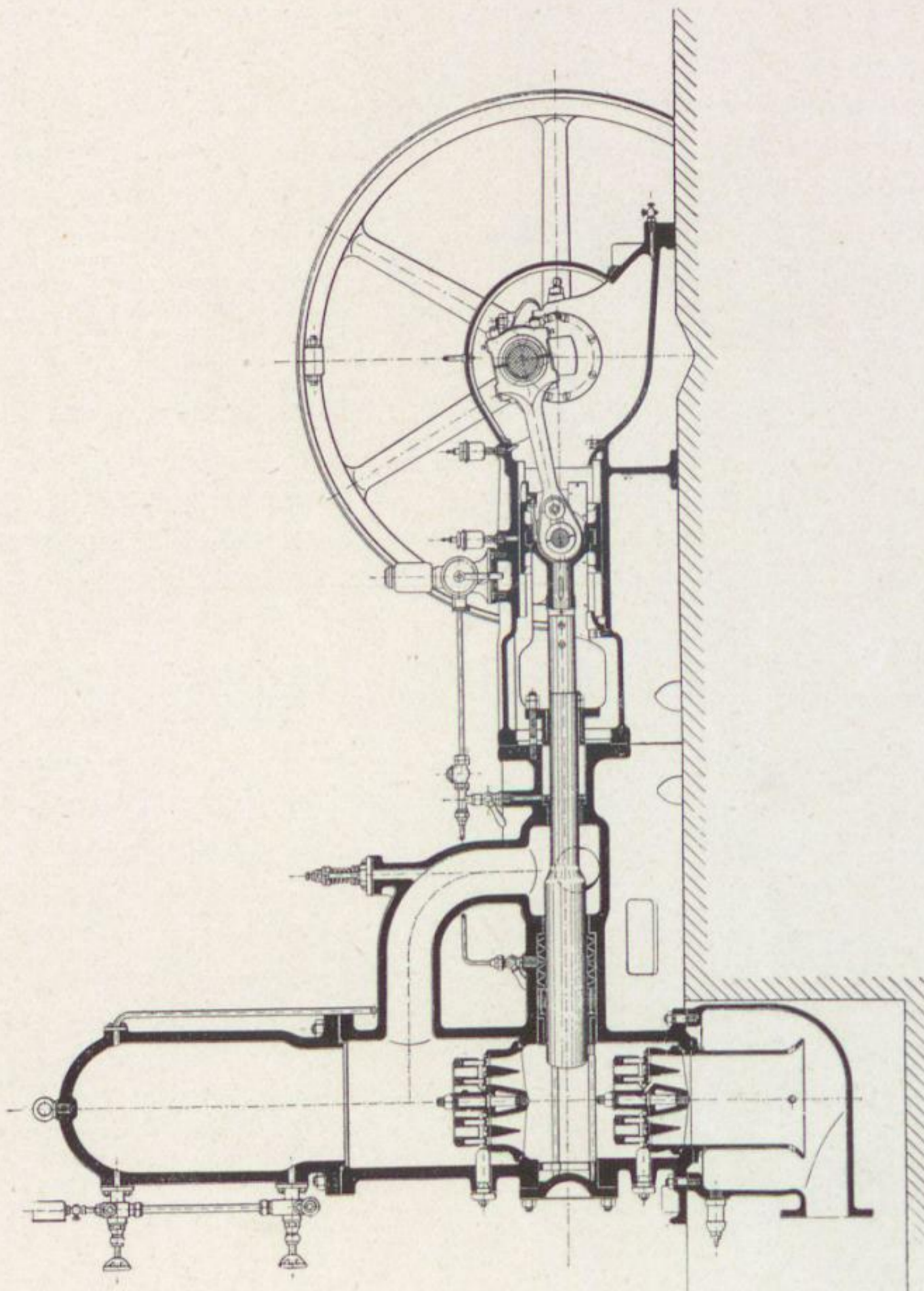
Schnellaufende Stufenplungerpumpe mit Innenstopfbüchsen für hohen Druck.
