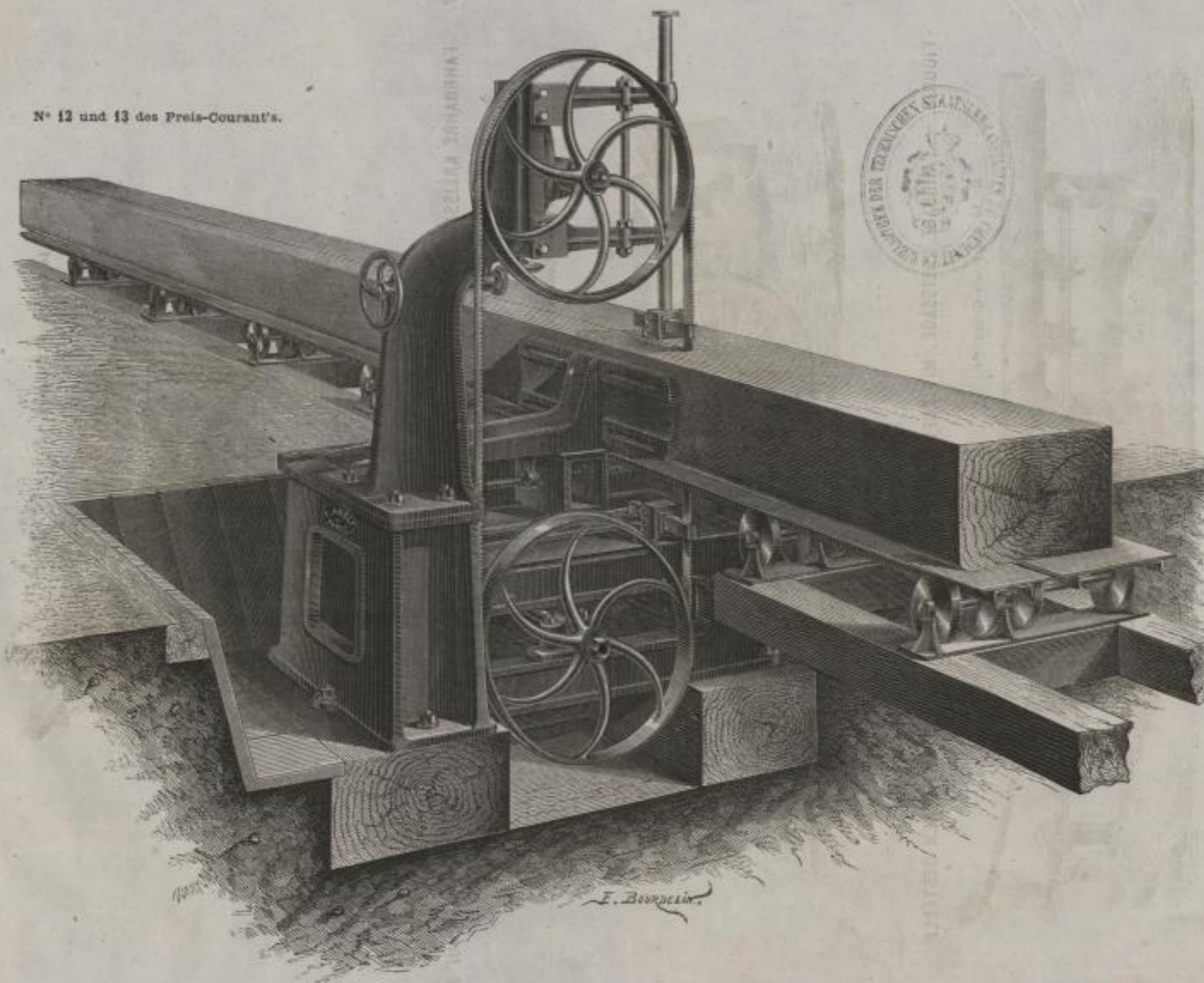
FIGUR 5. — BANDSÄGE; DER LÄNGE NACH GETHEILTER WAGEN, BAND DURCH DIE MITTE DES WAGENS GEHEND
