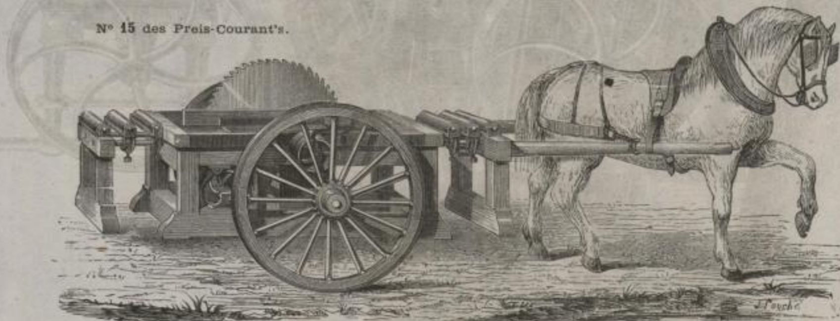
FIGUR 7. FAHRBAHRE KREISSÄGE, MIT ZUFUHRAPPARAT UND WALZEN AUF AUSZIEHBAREM GESTELL. FAHRBAR AUF RÄDERN DURCHMESSER DES BLATTES BIS ZU 1.20 M.
