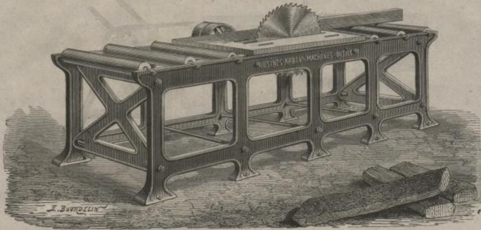
FIGUR 16. — KREISSÄGE MIT VERSTELLBARER AXE ZUM FALZEN, NUTHEN, ABSCHRÄGEN UND QUERSCHNEIDEN; GESTELL VON EISEN
