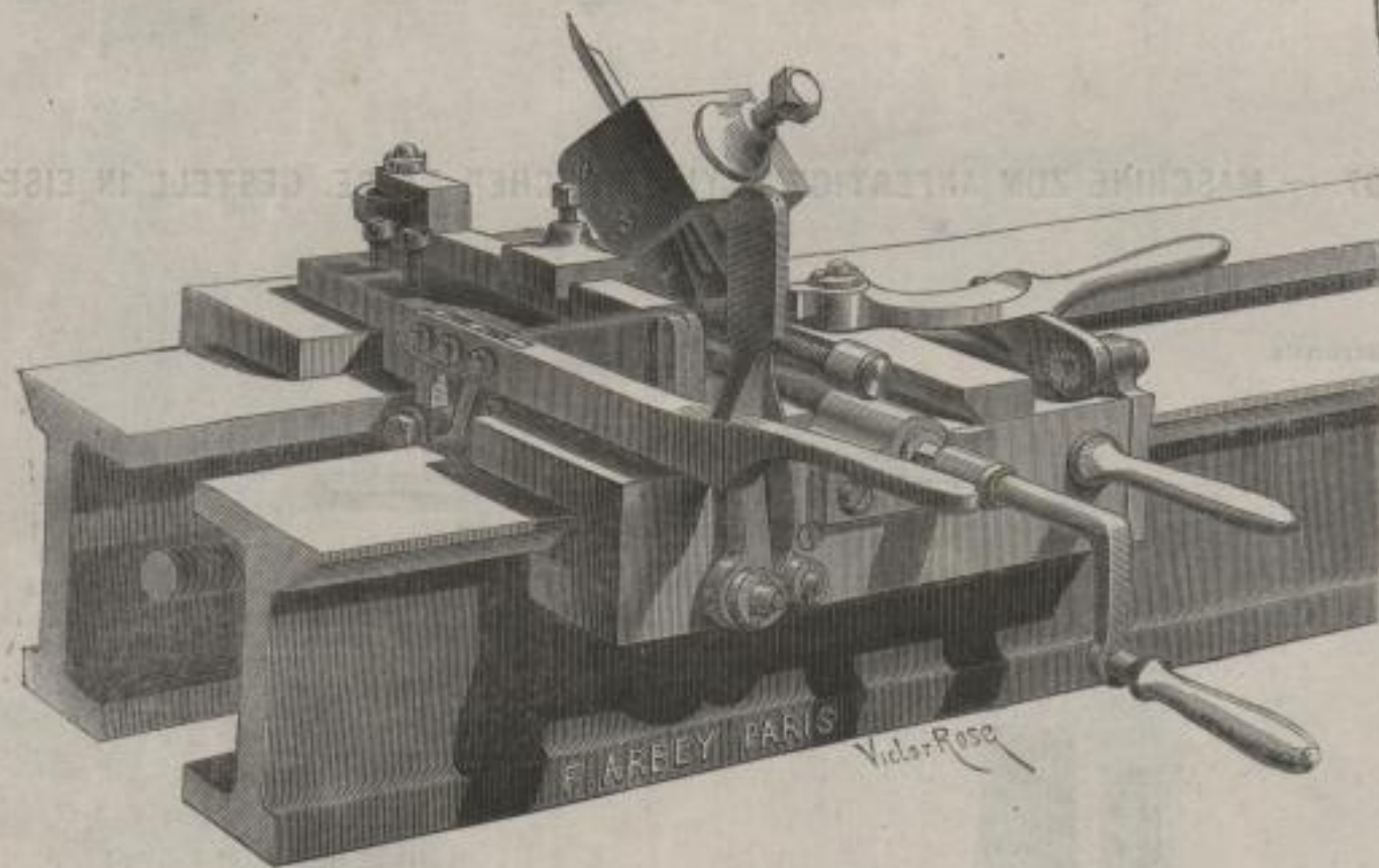
FIGUR 94. — SCHLITTEN DER SELBSTTHÄTIGEN FAÇONDREHBANK
