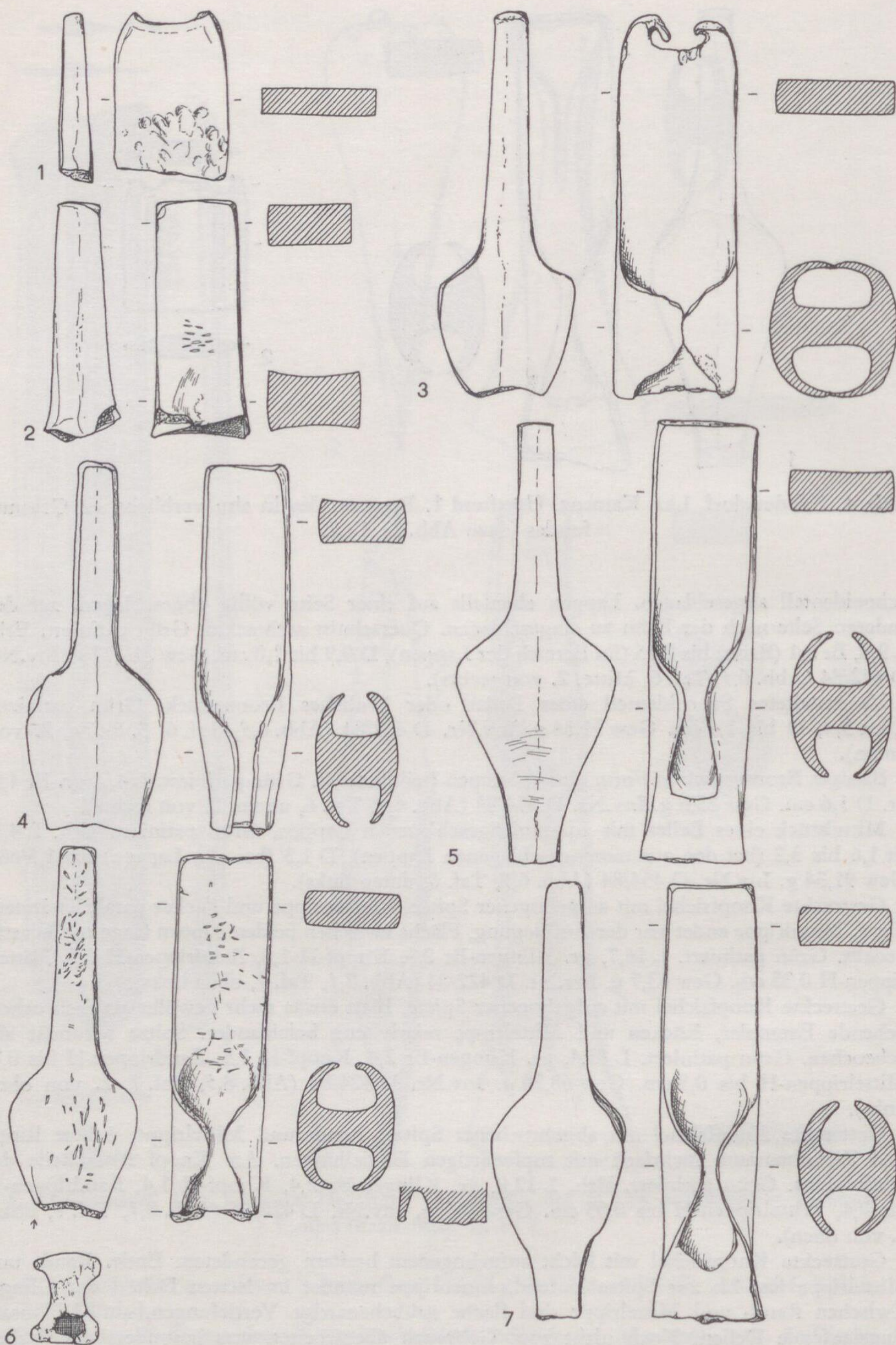
Abb. 5. Friedersdorf, Lkr. Kamenz. Hortfund 1. Bruchstücke mittelständiger Lappenbeile. 1:2.
