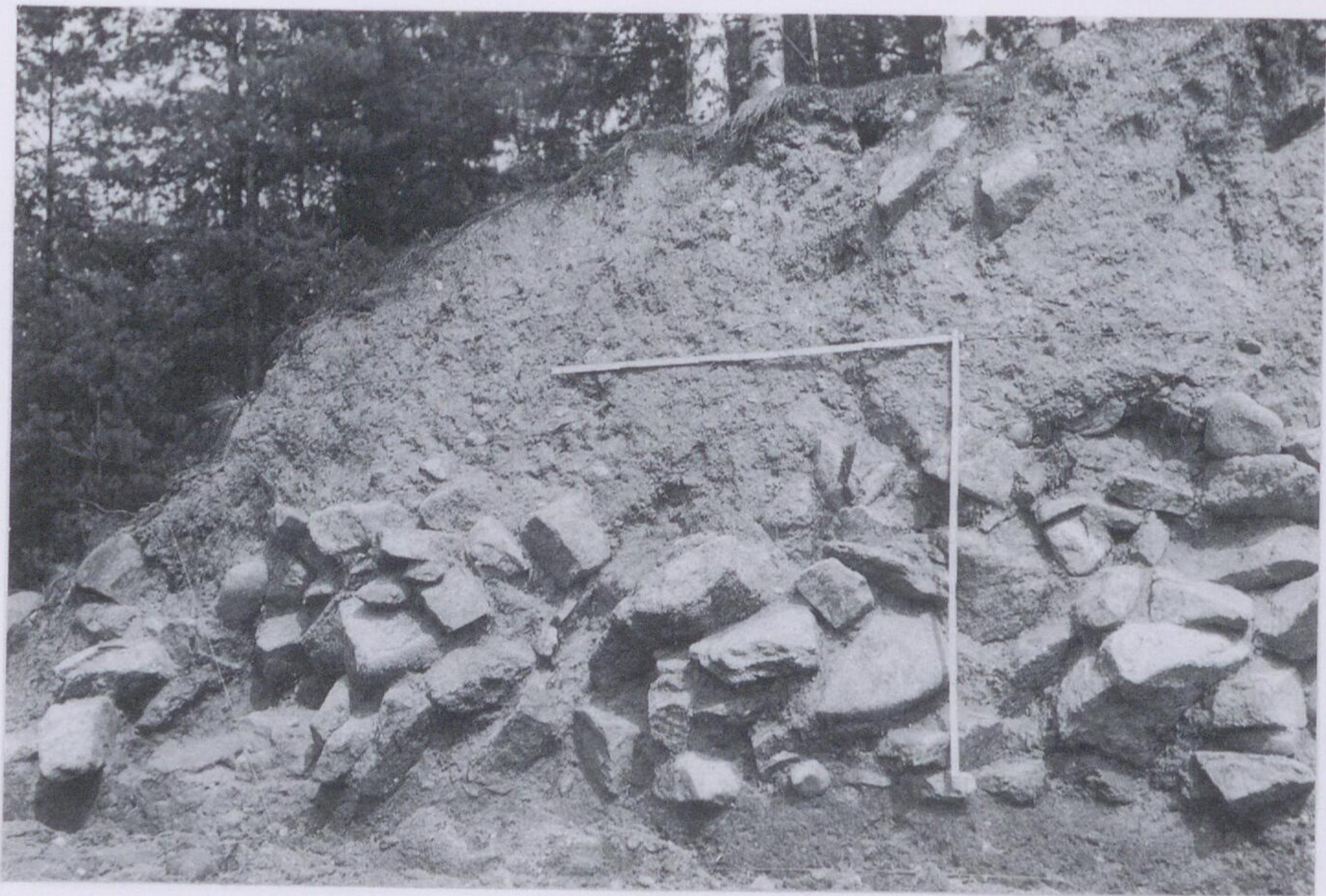
Tafel 2. Horka, Lkr. Kamenz. Hügel 1, a Resthügel von Nordwest mit Blick auf Nordteil von Profil 2; b Nordteil von Profil 2.
