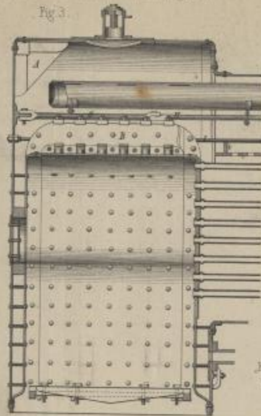
Feuerkasten der Locomotive „Liverpool“ nach Crampton's System.
