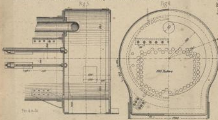
Rauchkammer von Tenderlocomotiven der Bergisch-Märkischen-Eisenbahn
