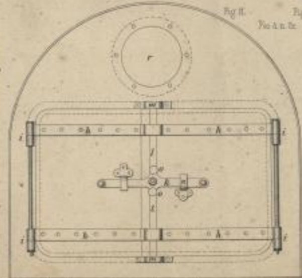
Rauchkammer-Thürverschluss von Heusinger von Walberg
