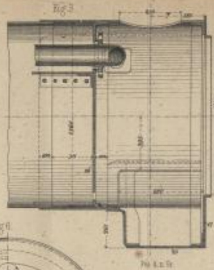
Rauchkammer von Tenderlocomotiven der Bergisch-Märkischen-Eisenbahn
