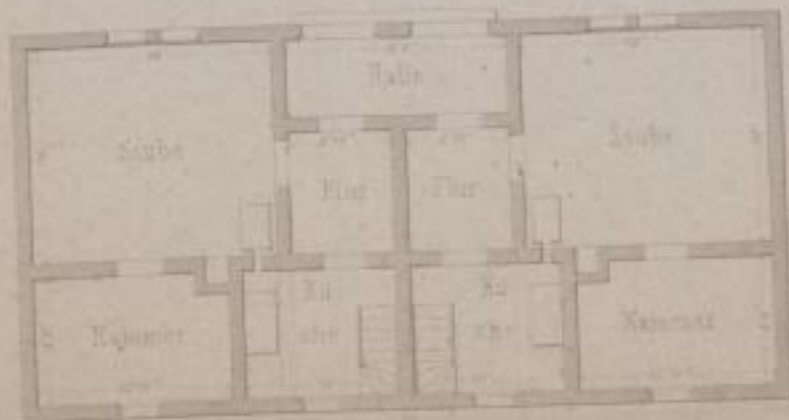
Grundriß
