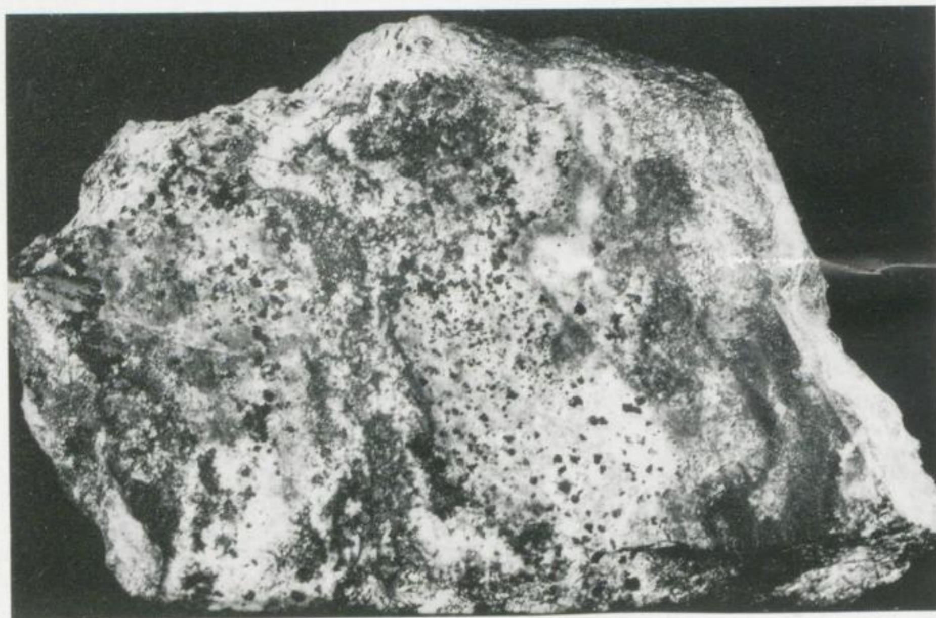
Bild 2. 1 Gangbezirk Kleinvoigtsberg („Alte Hoffnung Gottes“), Heinrich Sth., 11. Gez. Str. Feinkörnige Gangtextur des „eq-Typs“. Die Erzminerale (Sulfide und Silberminerale) liegen bevorzugt als fein- bis mittelkristalline Einsprenglinge innerhalb einer Quarz-Karbonatgrundmasse. M. 1 : 1,4
