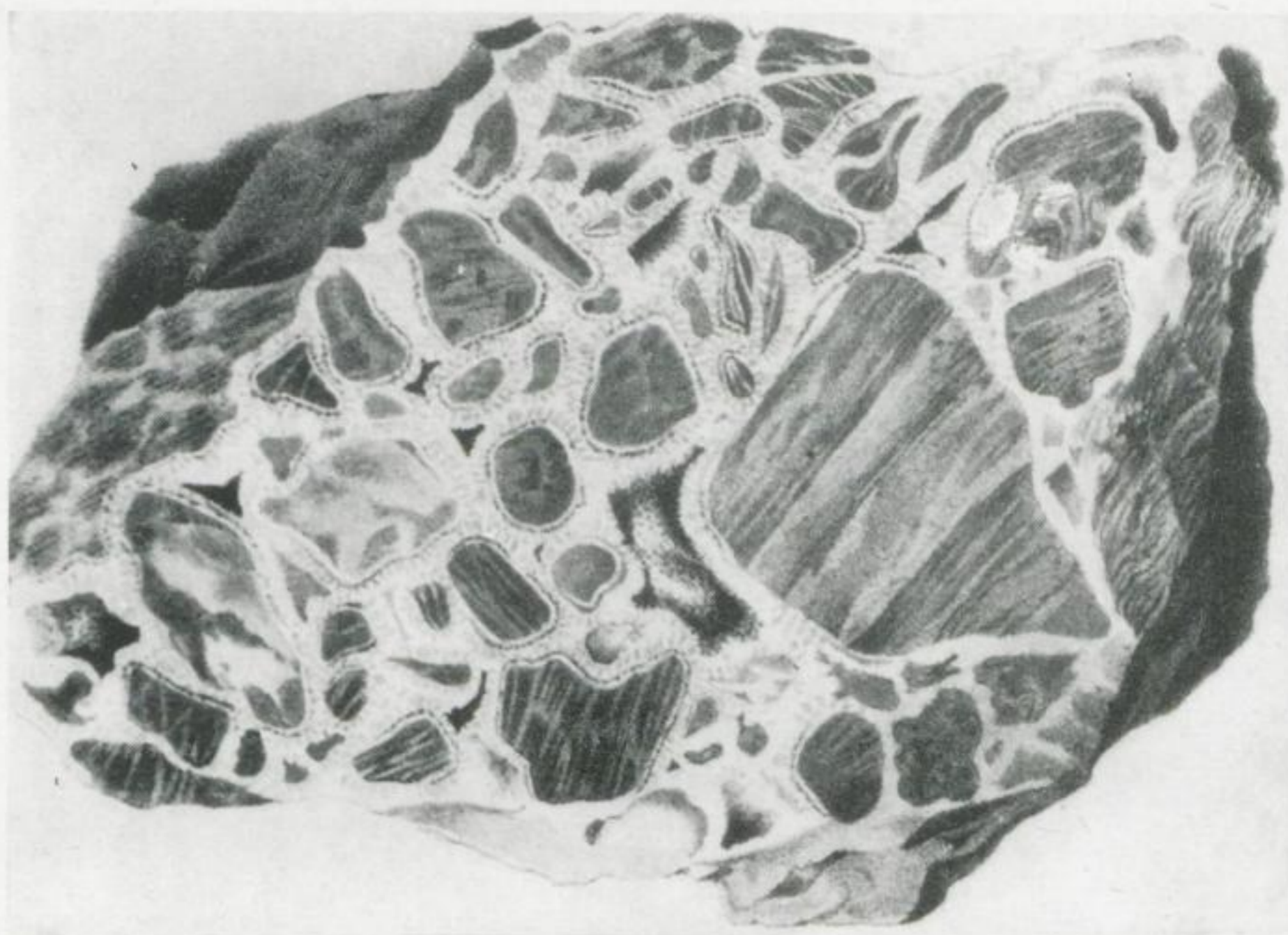
Bild 3. Gangbezirk Kleinvoigtsberg („Christbescherung“), Peter Sth. Sog. „Sphärogesteine“ (aus Weissenbach , 1836): Glimmerschieferbruchstücke werden von pyritführenden Quarzlagen konzentrisch umhüllt. In den Drusenräumen zwischen den „Sphären“ befinden sich oftmals Karbonate der eb-Formation (Manganspat, Braunspat). M. 1 : 2
