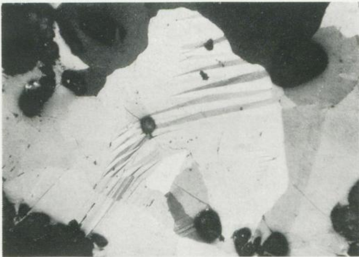
Bild 24. (Schliff Nr. 93) Gangbezirk Bräunsdorf („Glücksonne“ bei Mobendorf), Unbenannter Mg. Antimonit mit deutlicher Zwillingslamellierung. Vergr. 48 : 1, N +
