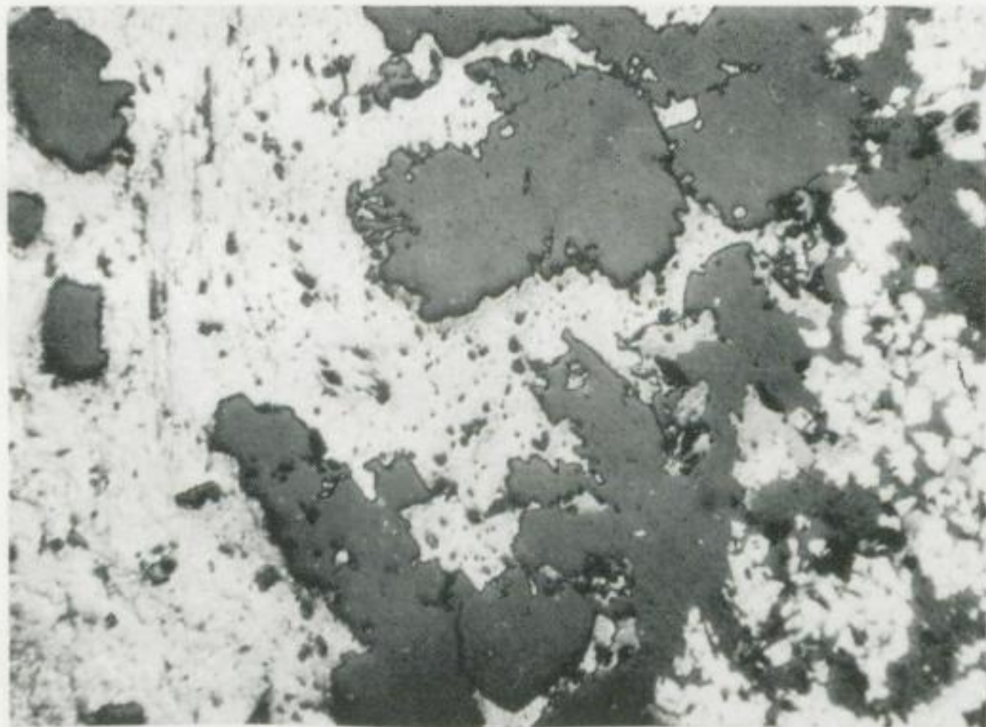
Bild 25. (Schliff Nr. 215) Gangbezirk Kleinvoigtsberg („Alte Hoffnung Gottes“), Beständigkeit Mg., 2. Gez. Str. Antimonit (weiß, porig) korrodiert intensiv älteren Quarz I + II. Im Quarz I feinkristalline Einschlüsse von „Tressenerz“ und Zinkblende I. Vergr. 48 : 1
