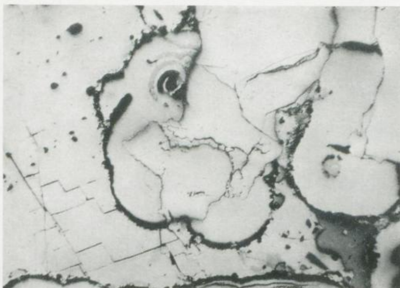
Bild 34. (Schliff Nr. 24) Gangbezirk Lichtenberg („König August“ bei Randeck), Friedrich Sp., \frac{1}{2} 2. Gez. Str.
