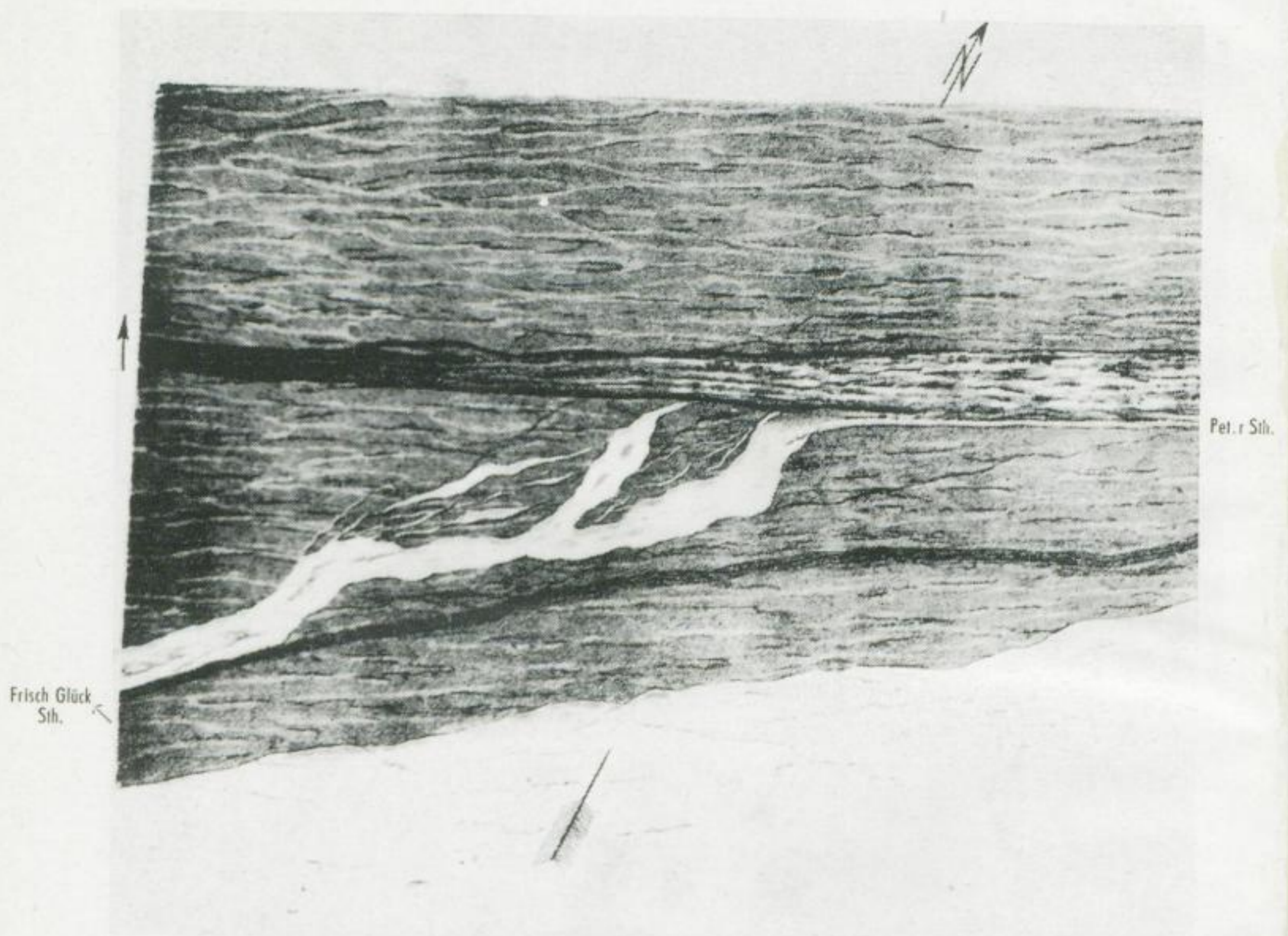
Bild 62. Gangbezirk Kleinvoigtsberg („Alte Hoffnung Gottes“). Anscharung des Frisch Glück Sth. an den Peter Sth., 3. Gez. Str. (aus Weissenbach , 1836). Beide Gänge zeigen deutlich die für sie typischen tektonischen Struktureigenheiten (Peter Sth. = s_1 -Struktur, Frisch Glück Sth. = F_1 -Struktur). M. 1 : 24
