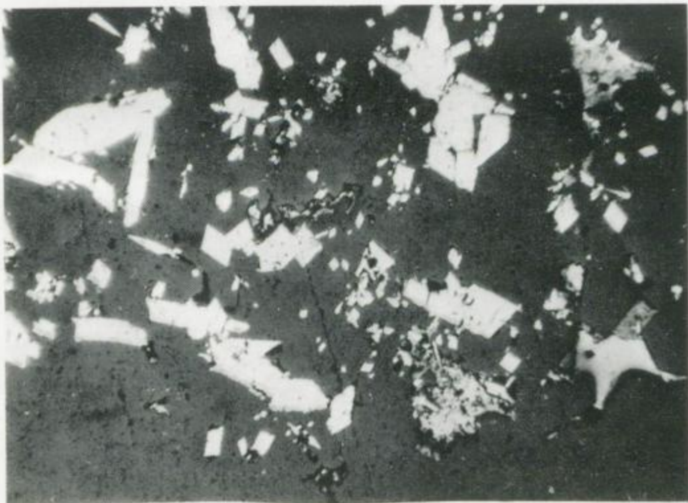
Bild 66. (Schliff Nr. 53b) Gangbezirk Siebenlehn („Vereinigt Feld“), Ludwig Sth., St.-S. Im Quarz I fein- bis mittelkristalliner Arsenkies (z. T. als „Tressenerz“). Als jüngere Zwickelfüllungen Tetradrit II und Pyrargyrit I (→ „Weißerz“- Bildung). Vergr. 48 : 1
