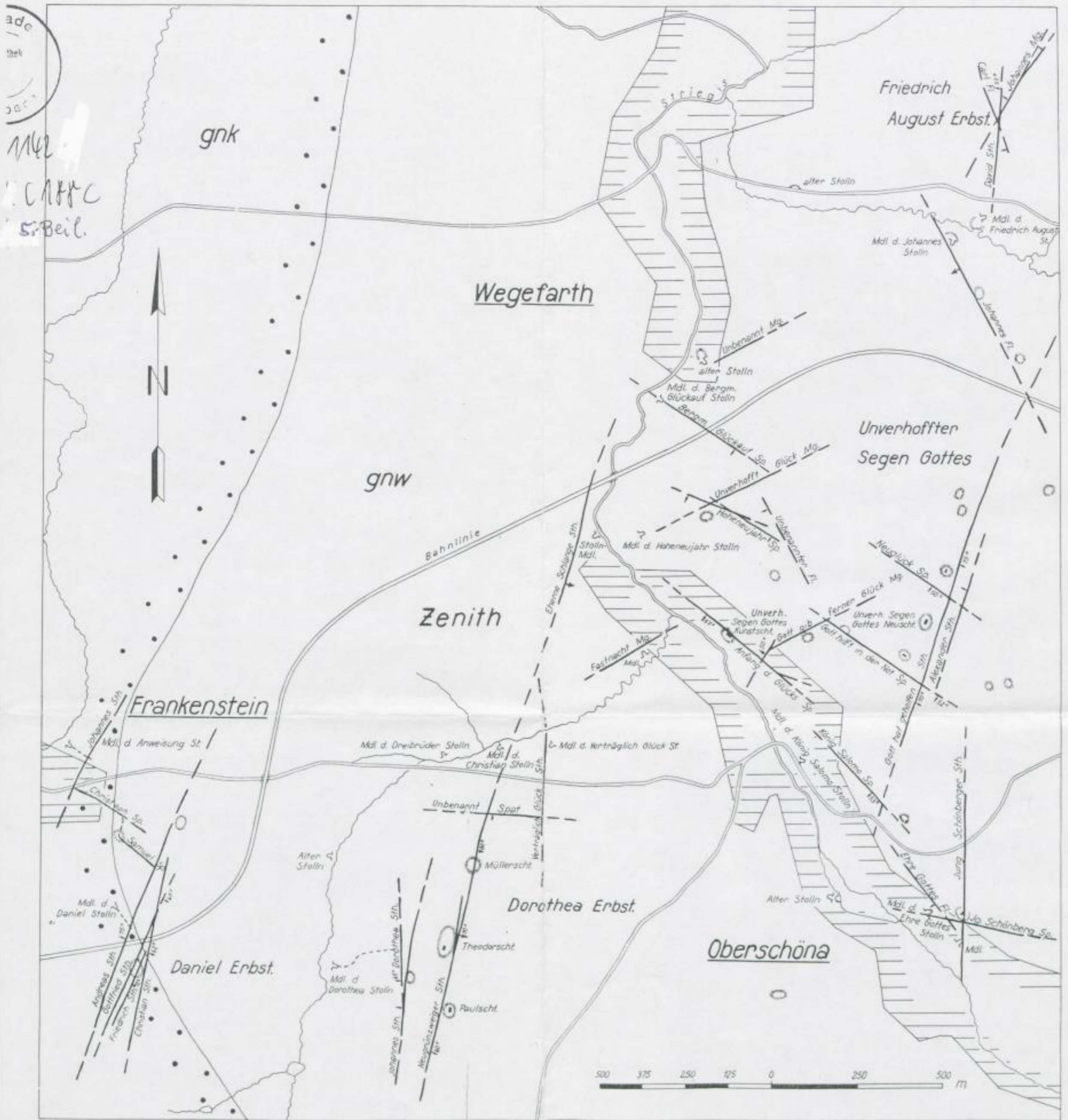
Bild 43. Geologie und Erzgänge des Gangbezirkes von Oberschöna (Teilgebiet)
