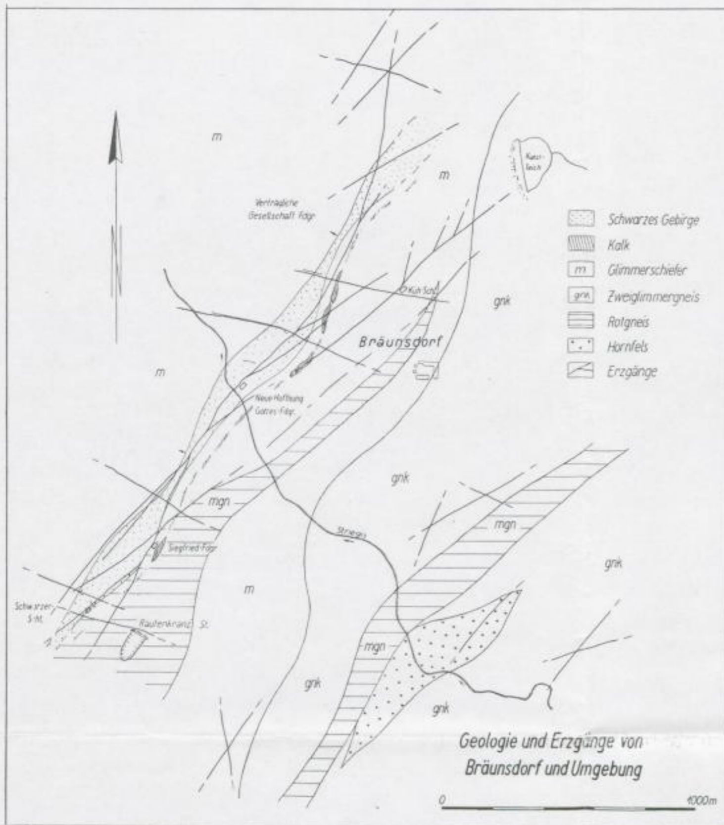
Bild 38. Geologie und Erzgänge von Bräunsdorf und Umgebung
