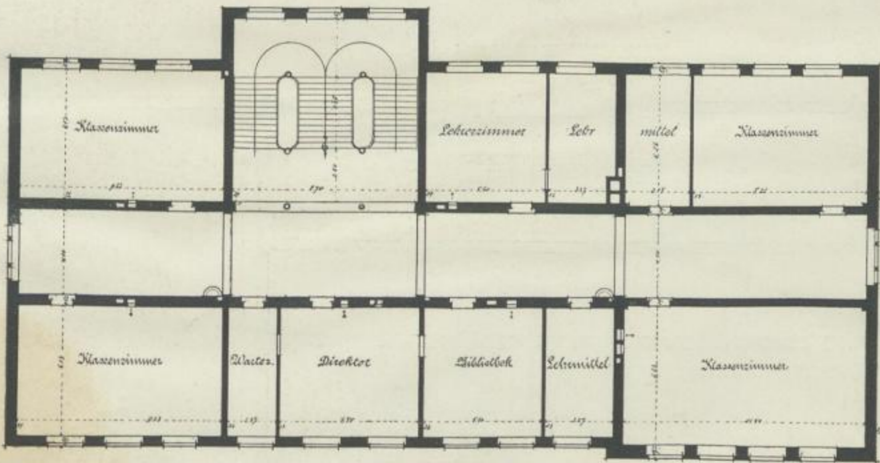
1. Obergeschoss
