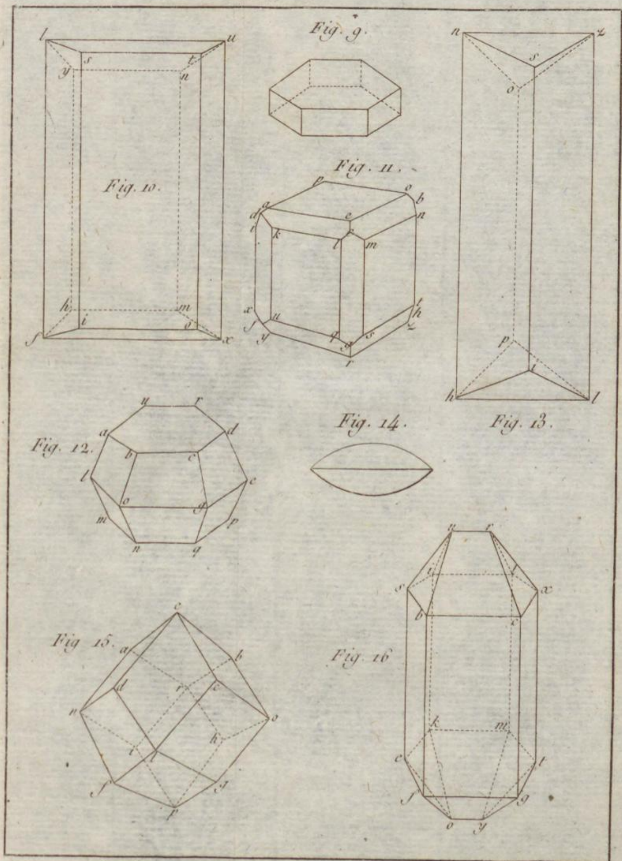
Fig 9. Spath calcaire en Table 10 et 13. Spath pesant cristallisé 11. Boracite. 12. Fer syntactique ou Mine de Fer spéculaire 14. Mine de Fer spathique 15. Grenat dodécaèdre à faces rhombes 16. Nitrate de Potasse.
