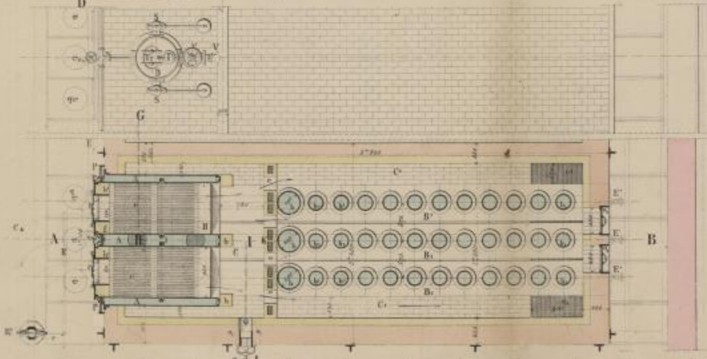
Fig 2 Ansicht von oben Schnitt nach EF.
