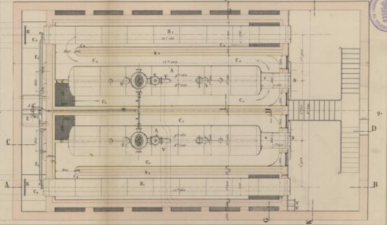
Fig. 2 Ansicht von oben - Schnitt nach EF
