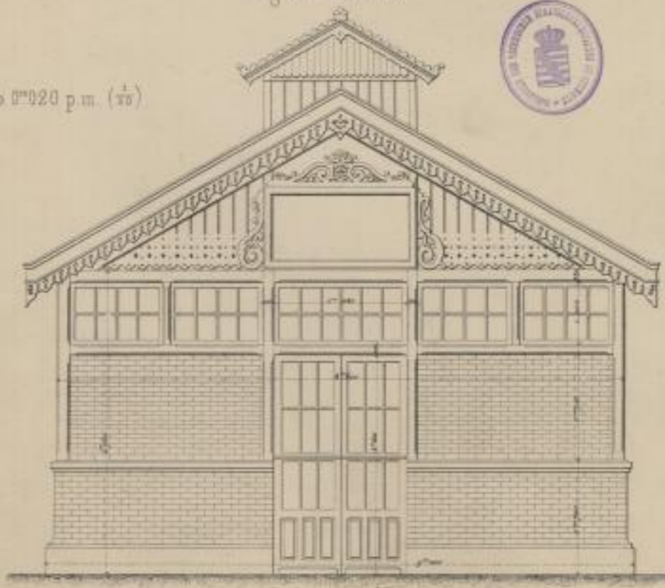
Fig. 6. Ansicht
