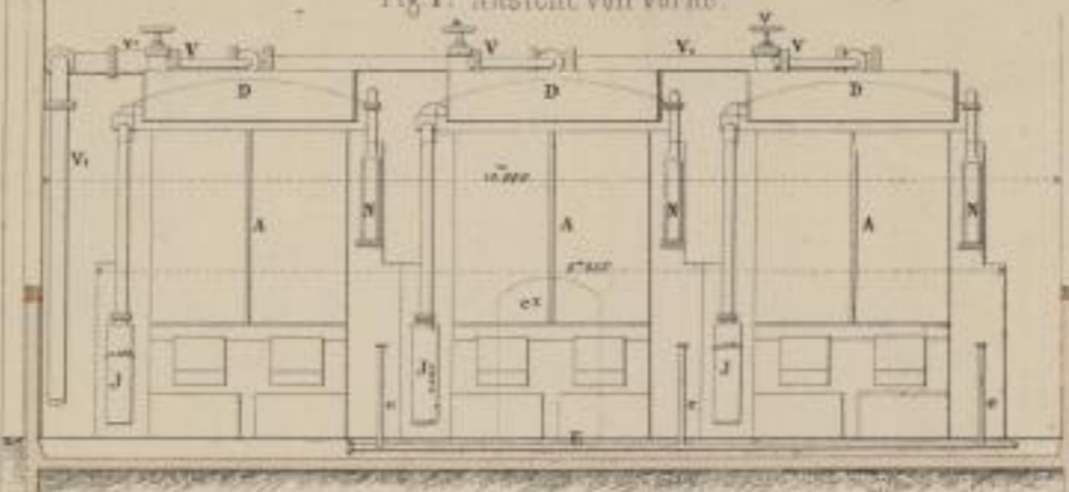
Fig 1. Ansicht von vorne
