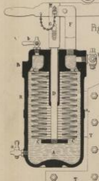
Fig 10 Schnitt nach AB
