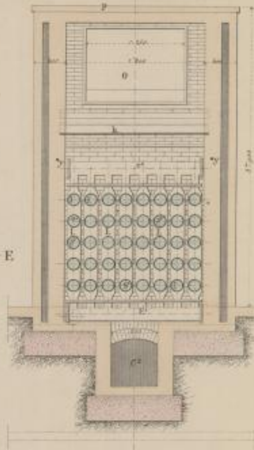
Fig. 4. Schnitt nach FG.
