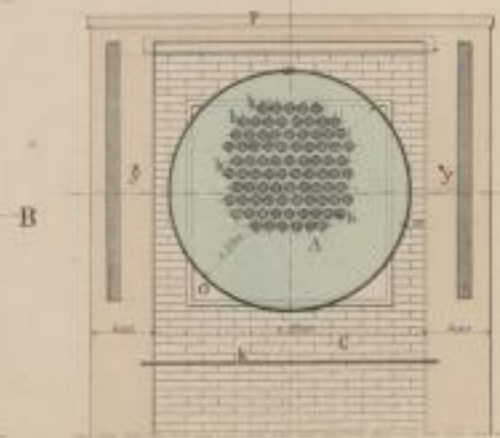
Fig. 4. Schnitt nach FG.
