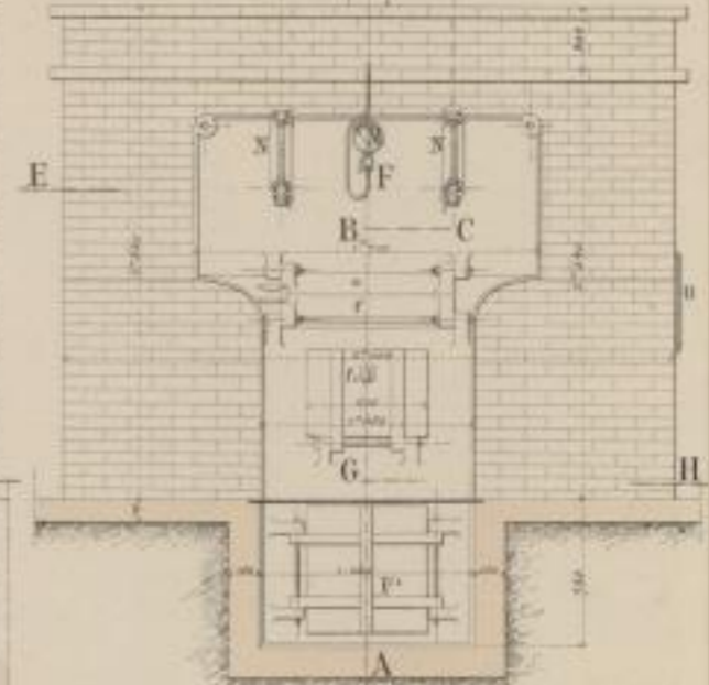
Fig 4. Schnitt nach IJ KL.
