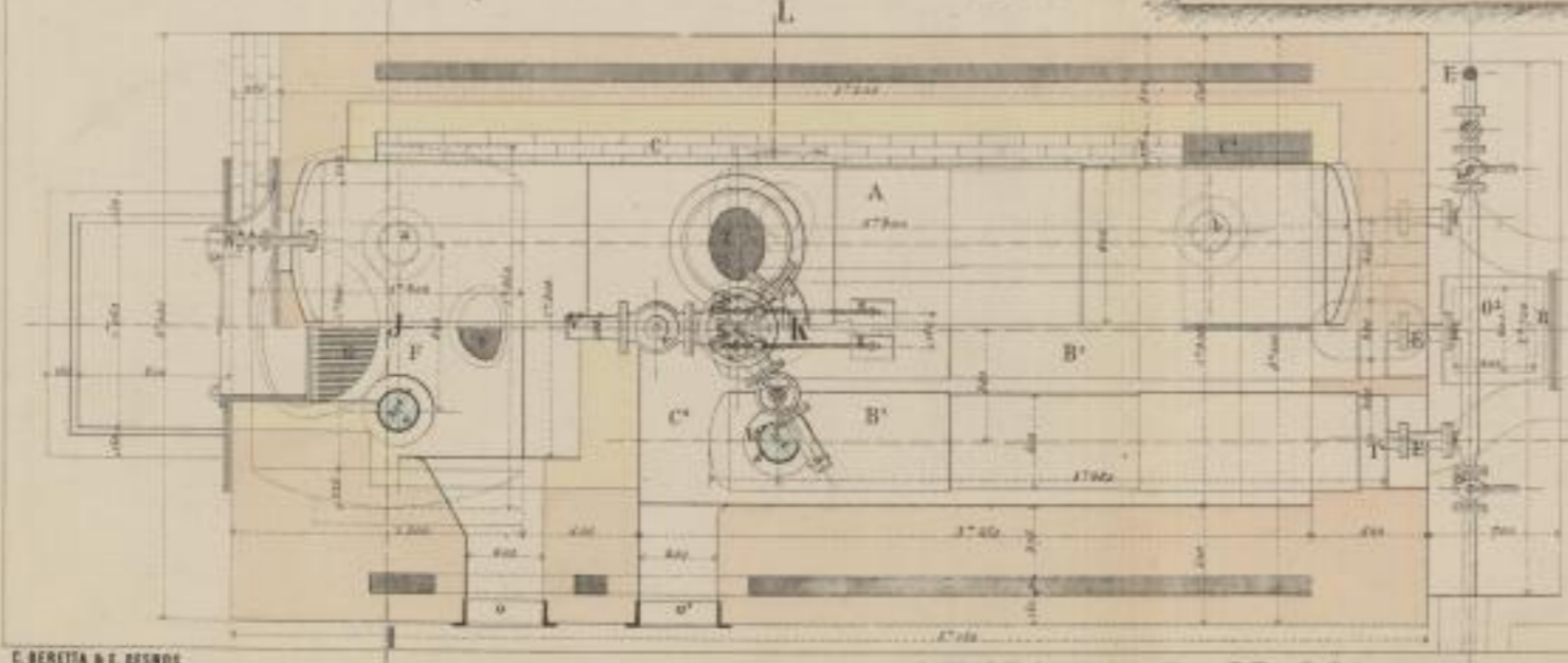
Fig 2 Ansicht von oben Schnitt nach EF.GH.
