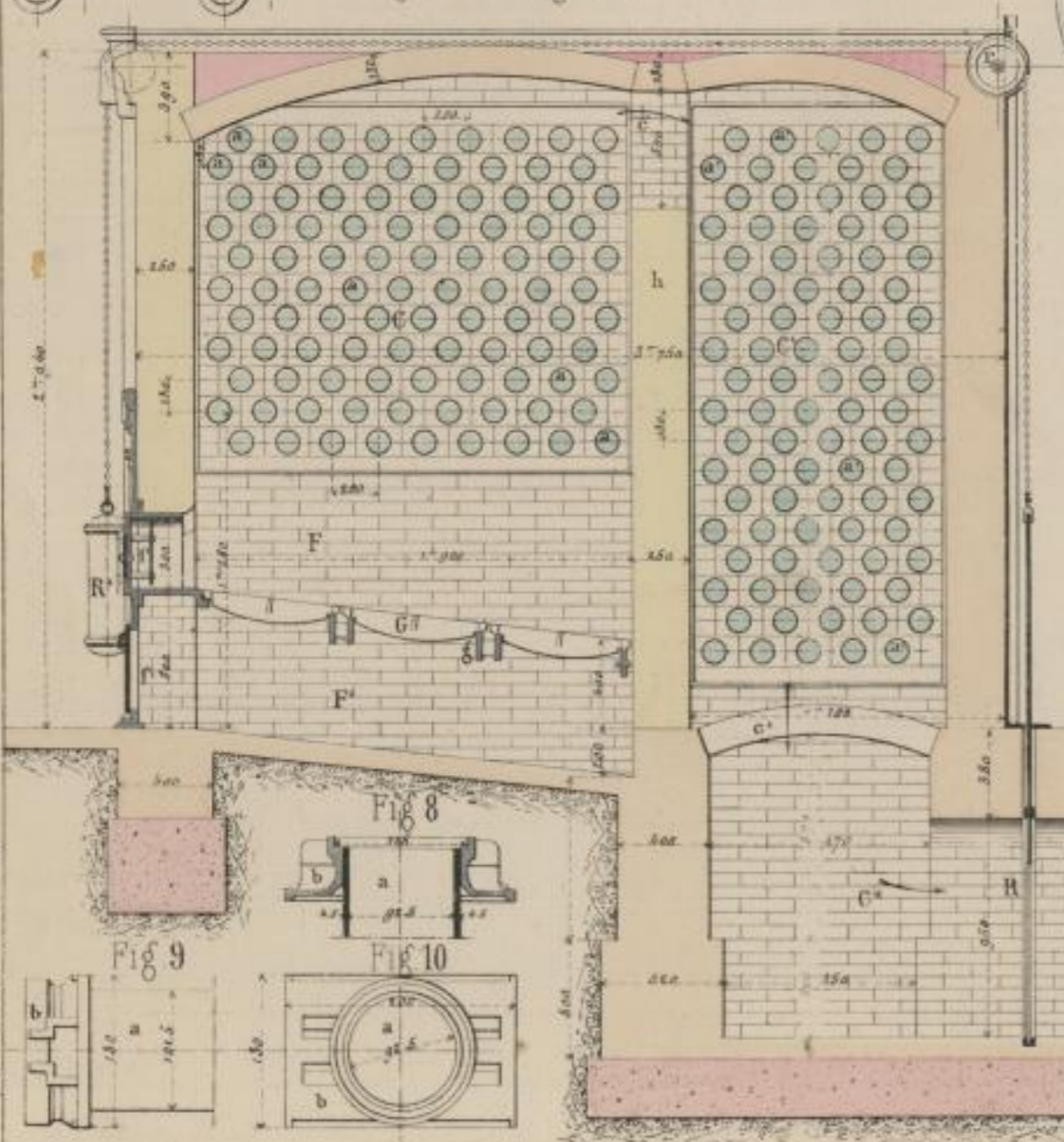
Fig 3. Laengenschnitt nach AB.
