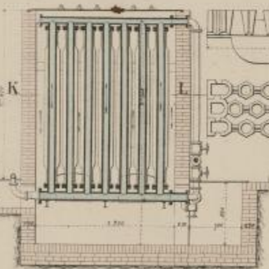
Fig. 10. Schnitt nach KL.
