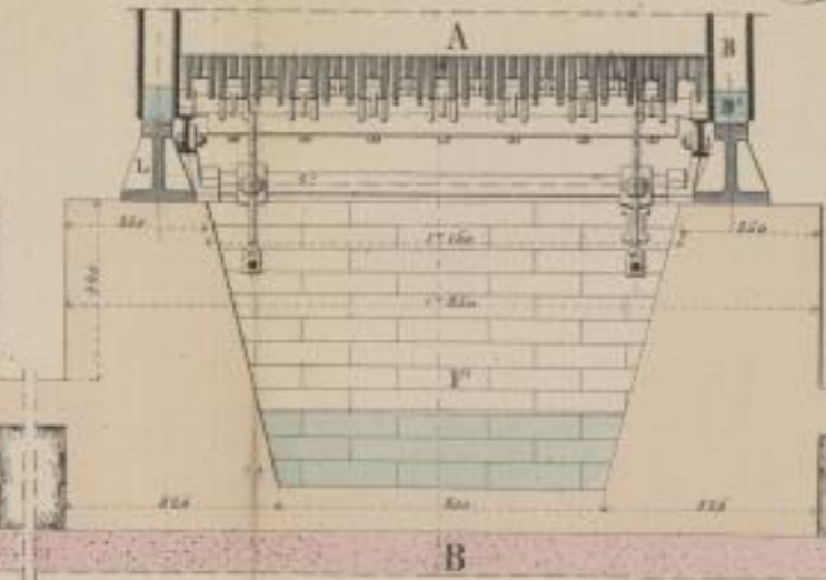
Fig. 2. Querschnitt nach CD.
