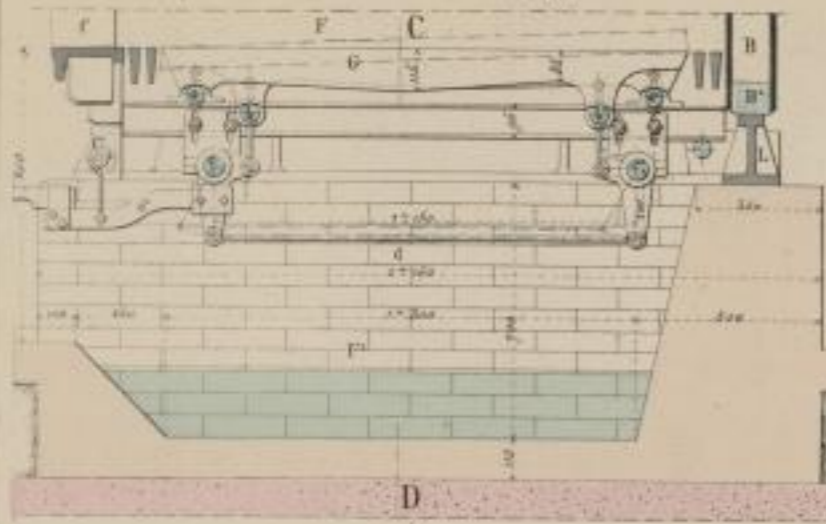
Fig. 1. Längsschnitt nach AB.
