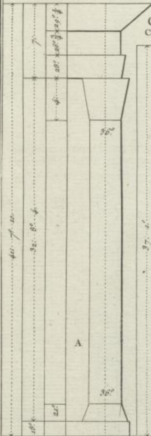
ORDRE Corinthien de la Nef de l'Oratoire.
