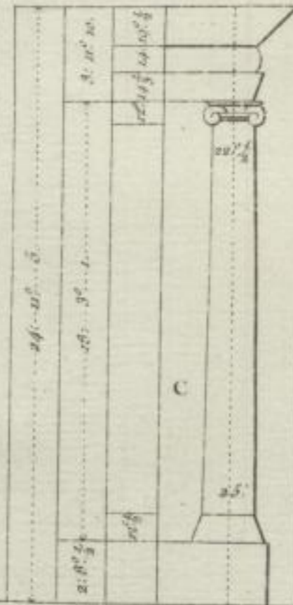
ORDRE Ionique du Portail de l'Annonciade a St. Denis.
