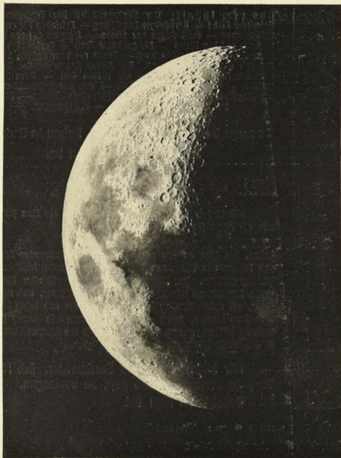
Der Mond im Alter von sechs Tagen. Umgekehrtes Bild, wie im astronomischen Fernrohr.
