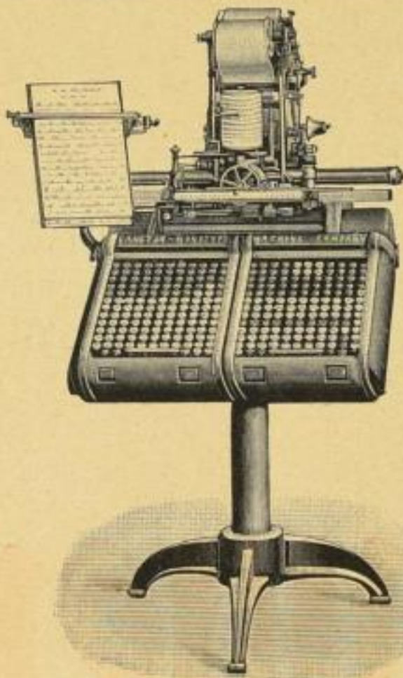
Neue Monotype-Setzmaschine mit Universal-Schreibmaschinen-Tastatur (Tastapparat Modell „D“)
