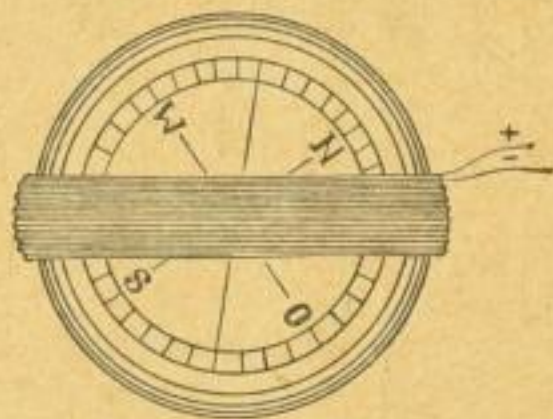
Abb. 41. Ein aus einem Kompaß hergestelltes Galvanoskop.
