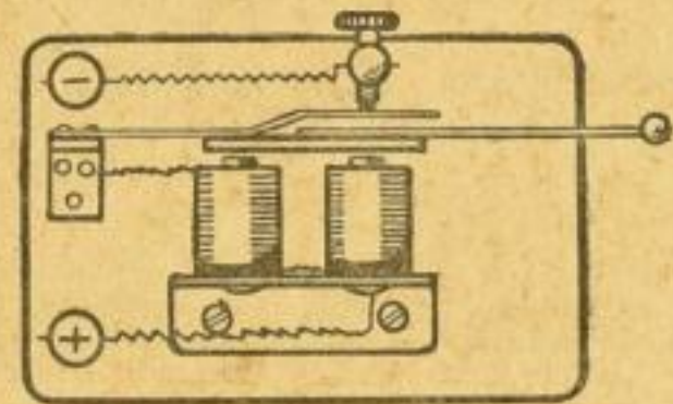
Abb. 75. Der aus einer alten elektrischen Klingel angefertigte Klopfer.
