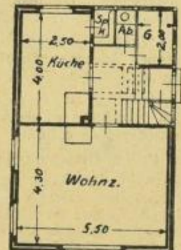
Abb. 17: Grundriss (Erdgesch.)
