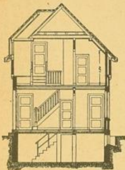
Abb. 70: Schnitt
