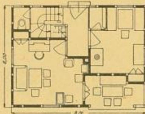
Abb. 53: Grundriß (Erdgeschoß)
