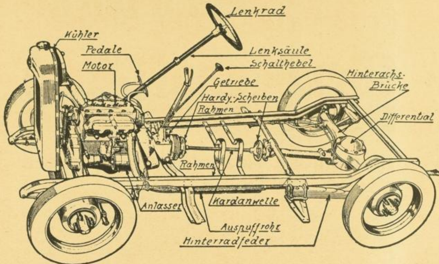
Abb. 3. Die wichtigsten Teile des Automobilchassis (halbschematisch).
