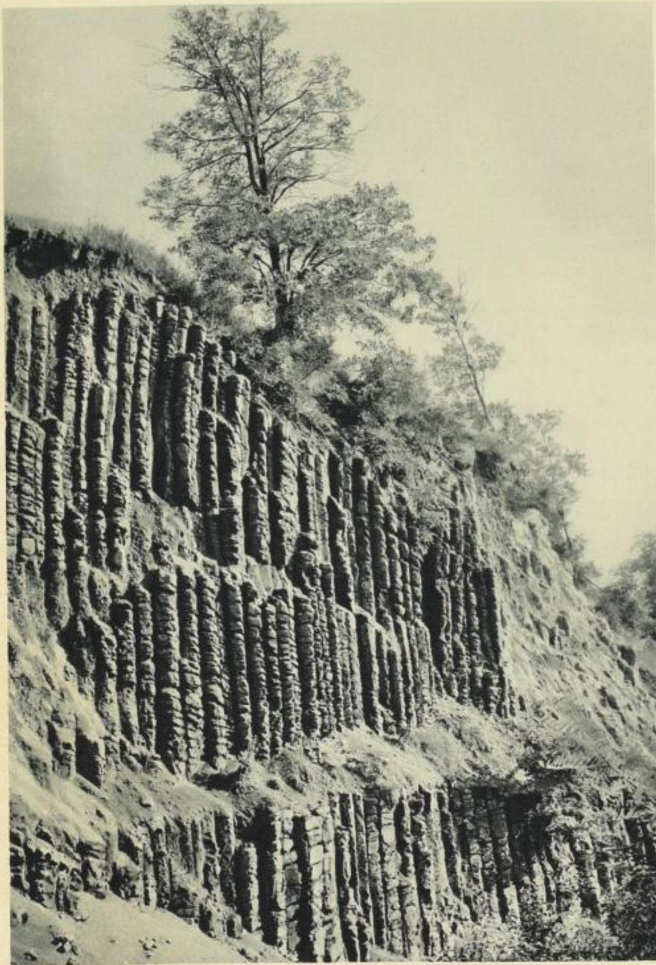
54. Säulenförmig absondeter Basalt bei Nikolstadt in Schlesien.
