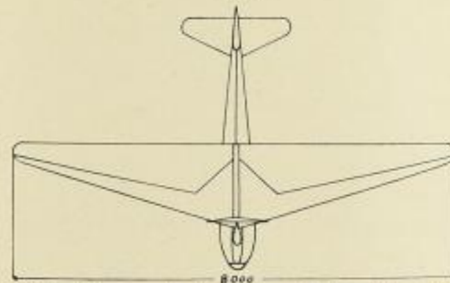
Muskelkraftflugzeug von Ing. Hoeffler, Dessau 1954. Zugschraubenantrieb
