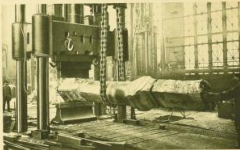
Nachschalle aus einem Stahlblock unter dem 100-Zentner-Hammer
