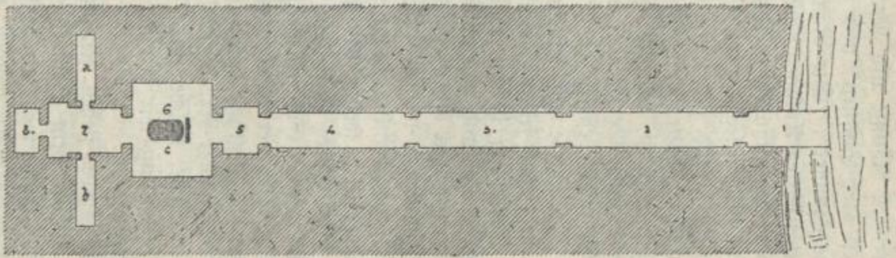
Ein Königsgrab aus dem Neuen Reiche. Horizontalburchschnitt.
