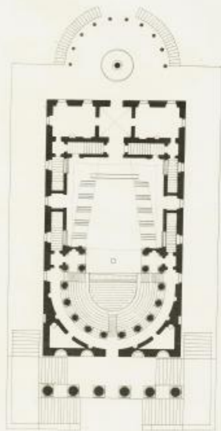
Ved. di Spitiach a Berge-Lan in Savoie. Piaz. di Quadrato disegnata per Luchini, in 1786.
