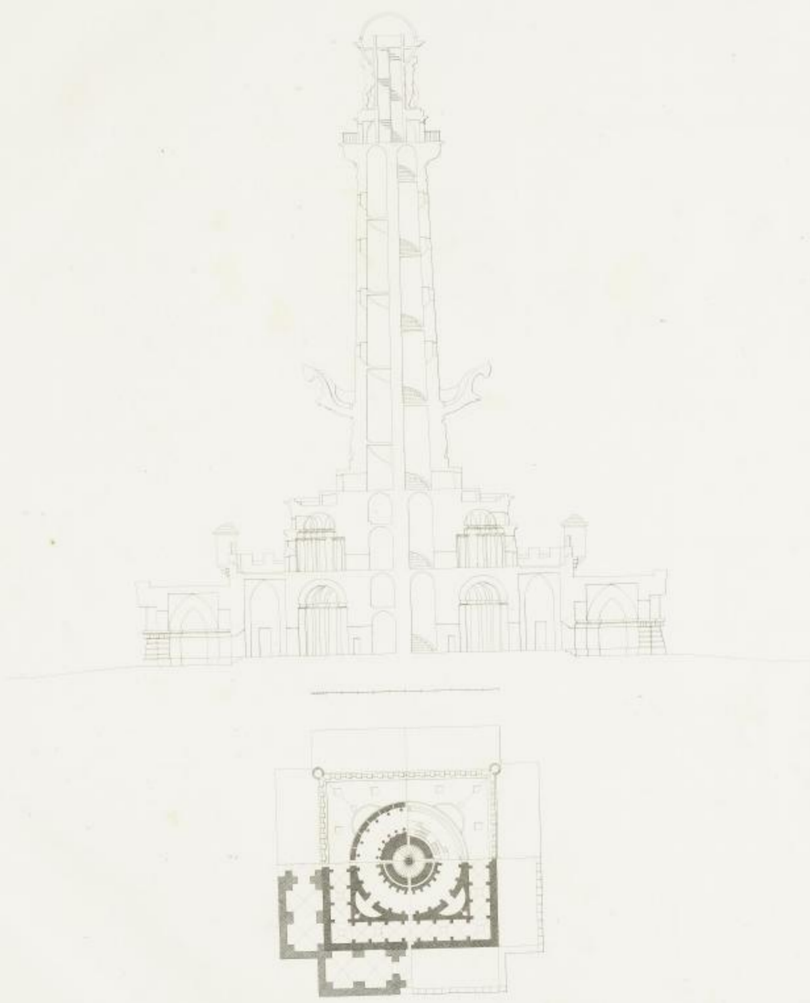
Plan et coupe de la colonne élevée par Harmand
