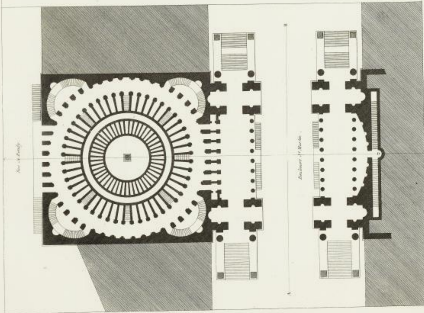
Projet d'édifice concertiste destinée à célébrer les fêtes nationales pendant l'hiver, dont l'un des projets par le Gouvernement, dans un concours public et remporté par Laboure en 1835. Plan N. de la République. Le local propose était l'ancien théâtre de l'épiscopi par St. Martin.
