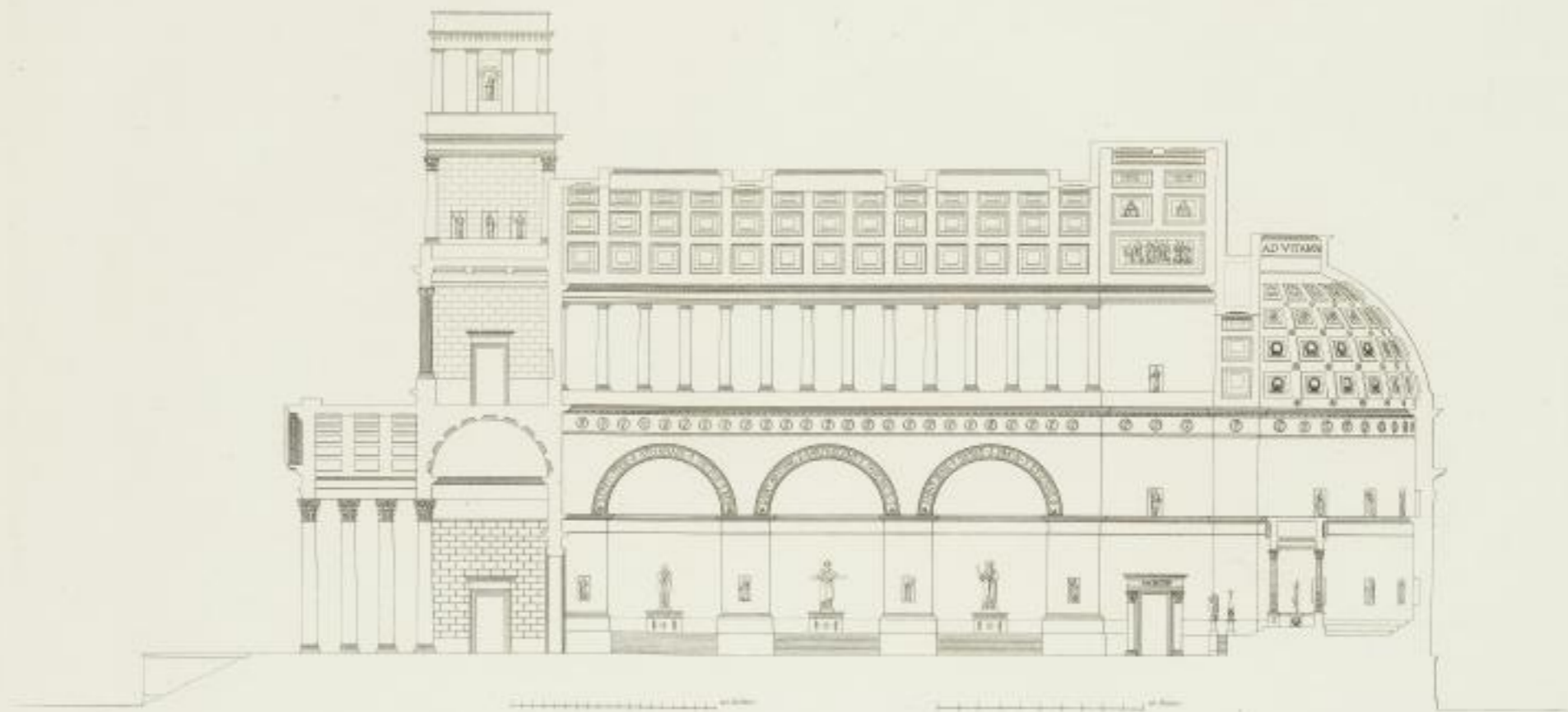
Coupe de la Basilique en Temple ancien par L'abbé
