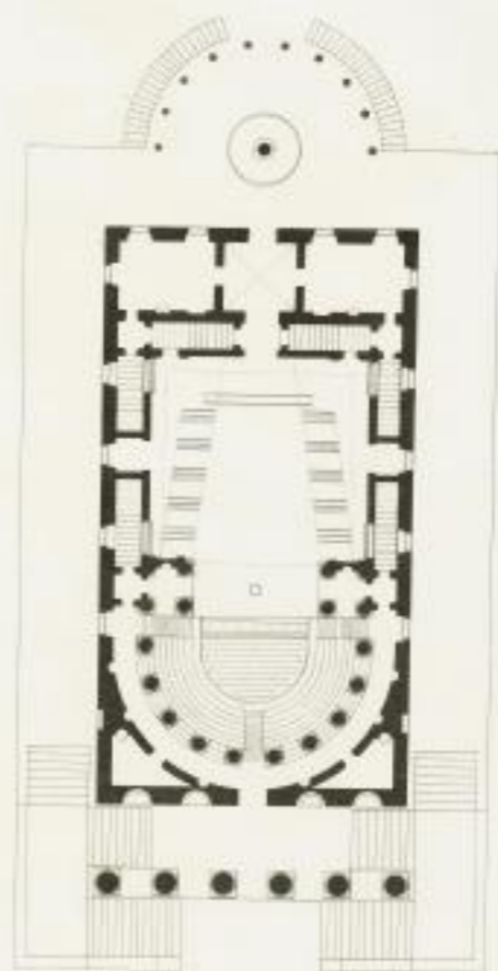
14. 1. Theater von Aspendos in Kleinasien. Von A. Brunn. Gezeichnet von Schuch, im Jahr 1841.
