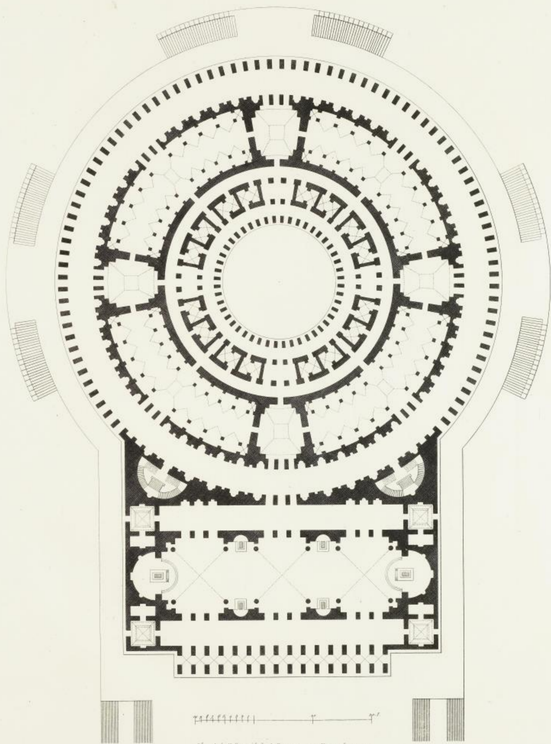
Plan de la Halle sur le bord d'une gare par Seroux, en 1791.
