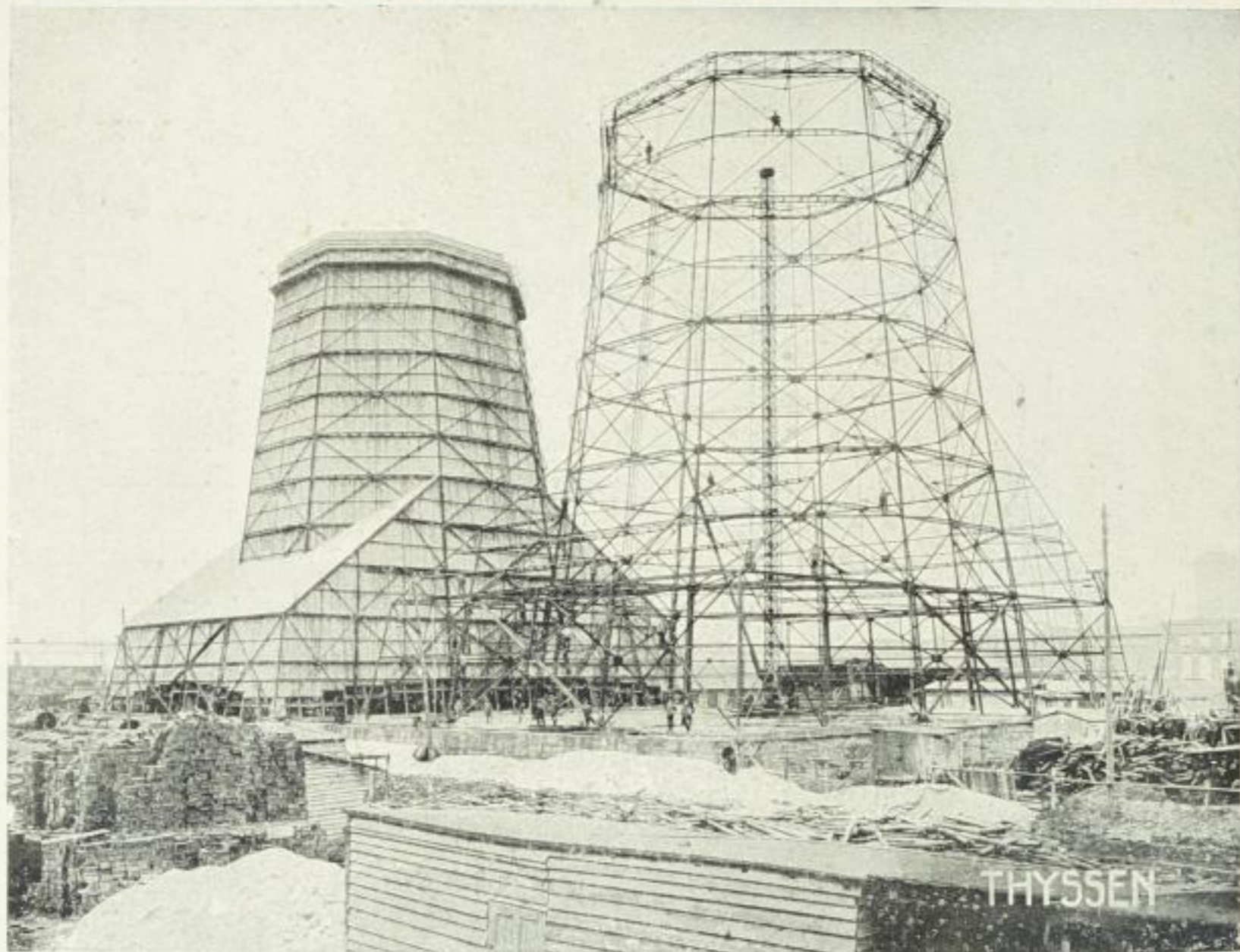
2 Thyssen-Zonenkühler im Bau, Gesamtleistung 16000 cbm/stdl.
