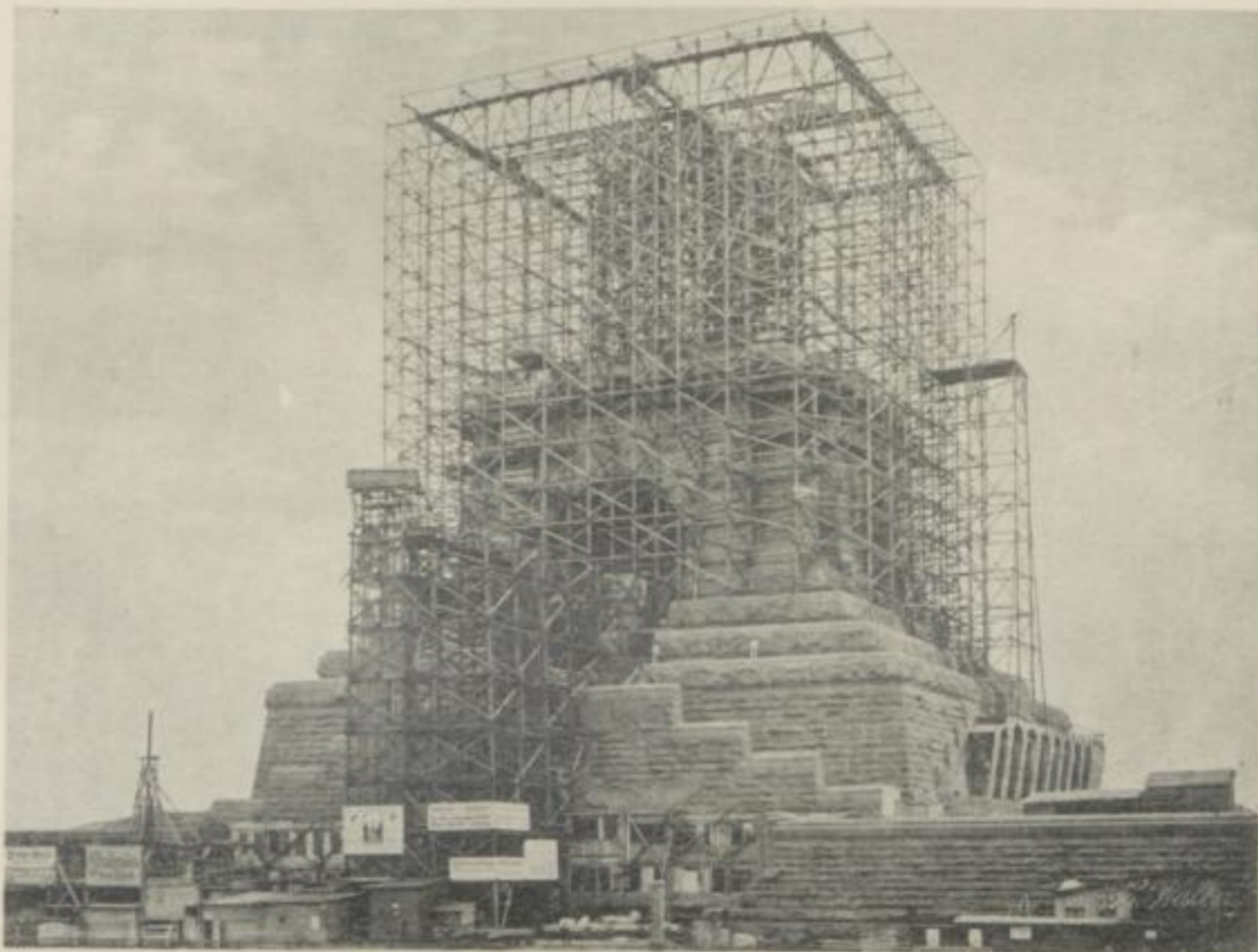
Vorderansicht des Denkmals in Höhe von 54 m (Juni 1909)
