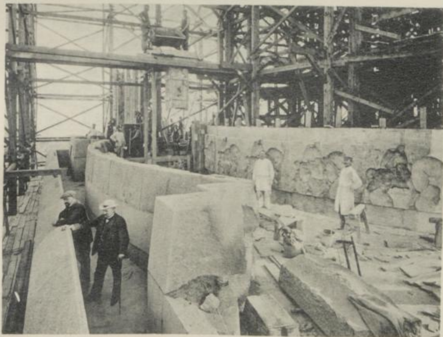
Blick auf den ersten Rundgang in Höhe von 57 m (September 1909)
